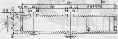
1-1剖面图
