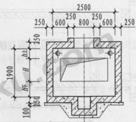
2-2剖面图
