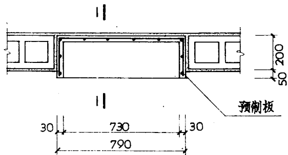
壁龛平面
