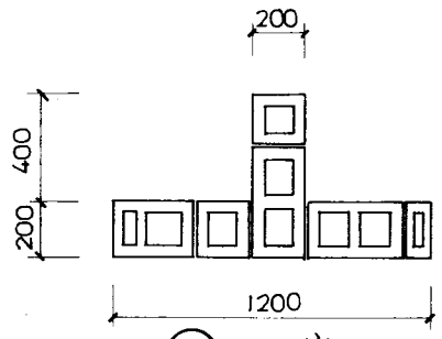
③ 三皮
