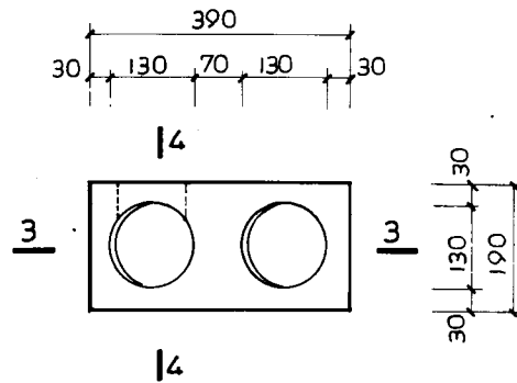
K 14 平面图
