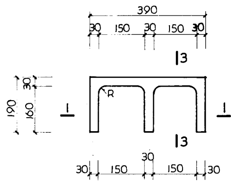
K 11 平面图
