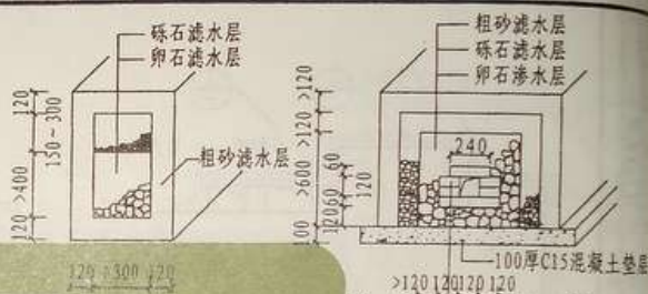
① 无管型
