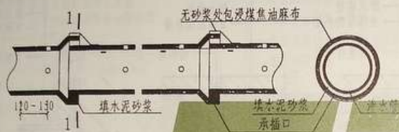
① 承插式 (一般管材 渗水管)
