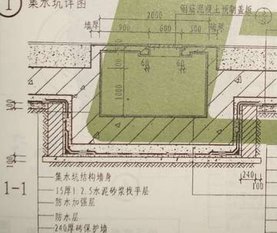
① 集水坑详图
