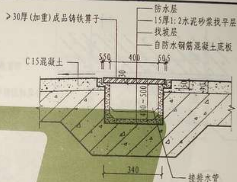
② 地下车库坡道截水沟详图
