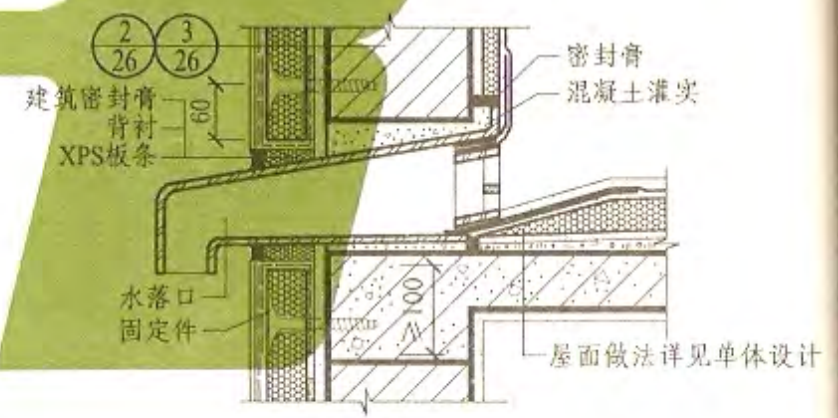
④ 水落口
