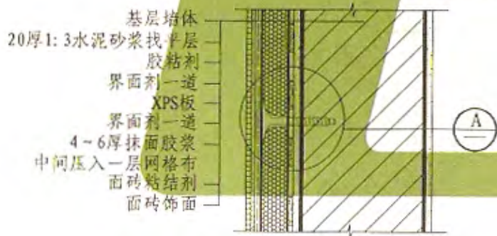
③ 面砖饰面系统
