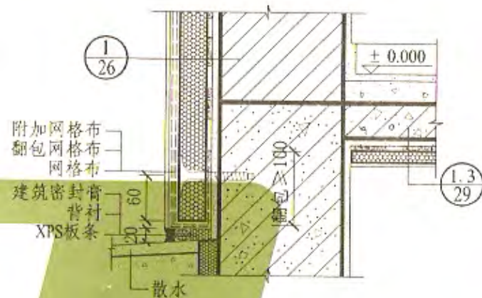
② 不采暖地下室外墙勒脚
