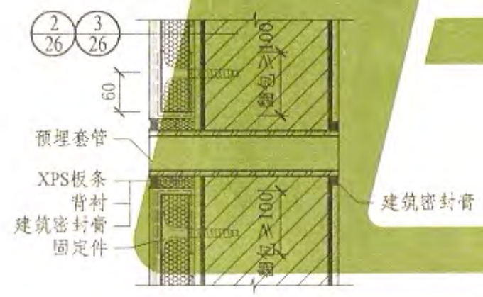
③ 穿墙管道
