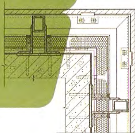
④ 幕墙阳角
