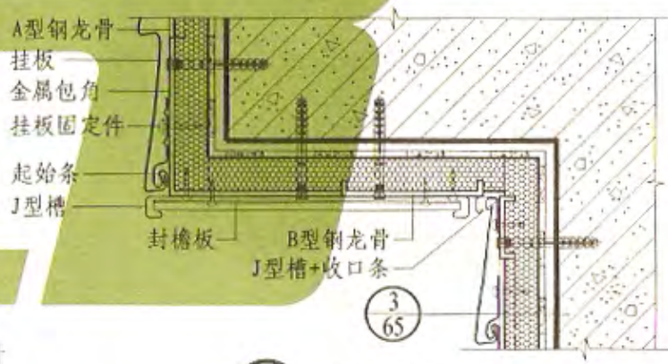
④ 外挑处挂板墙面构造
