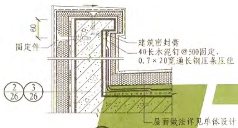
① 女儿墙
