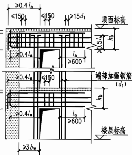
2 小墙肢处洞口连梁配筋示意
