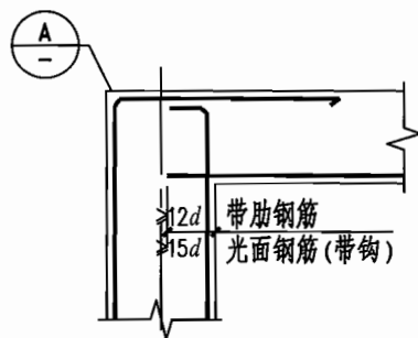
3e 顶层端节点 (用于计算不利用梁下部钢筋强度时)
