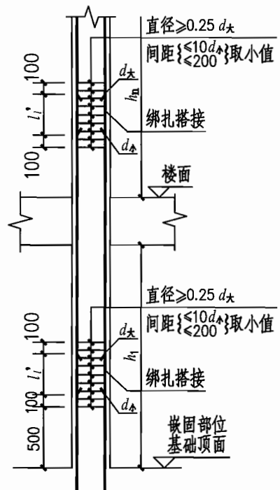
3 受压钢筋绑扎连接 d \leq 32 (接头外两个箍筋仅用于 d > 25 时)
