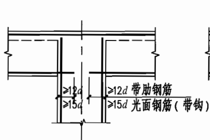
4c 顶层中间节点 (用于计算不利用 梁下部钢筋强度时)
