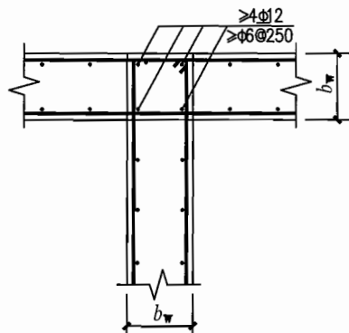
7 剪力墙端部配筋加强构造
