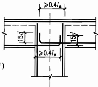
4d 顶层中间节点 (用于计算充分利用梁 下部钢筋受拉强度时)
