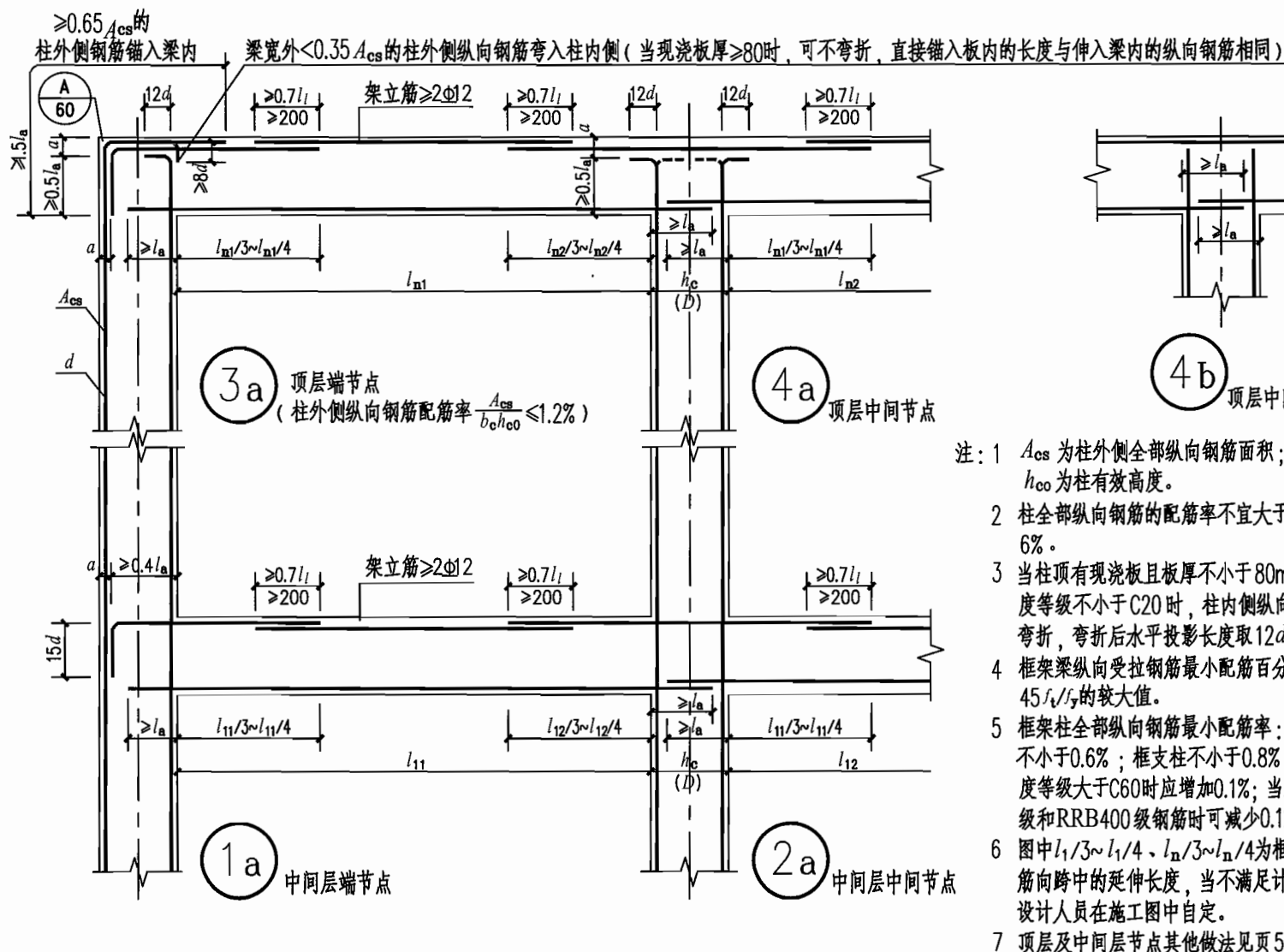
图 名 框架纵向钢筋构造 图集号 陕09G02 页 次 58
