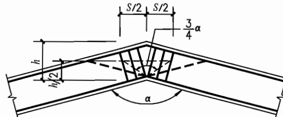
5 梁内折角处箍筋加强构造 (内折角处于受拉区时) S = h t g (3\alpha/8) (箍筋面积经计算确定)
