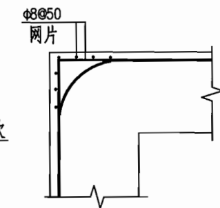
A (当有挑檐板、女儿墙或另向框架梁通过角部时可不设此网片)
