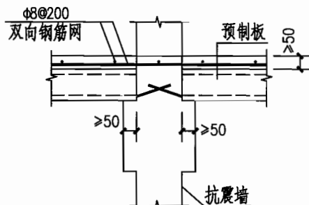
2 抗震墙边框架搁置预制板构造
