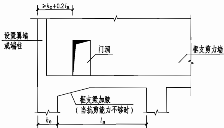
3 框支梁上墙体有门洞的构造措施
