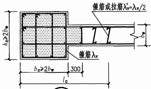
⑦ 有端柱
