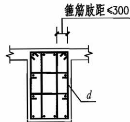
3 梁加密区箍筋肢距 (四级抗震等级)
