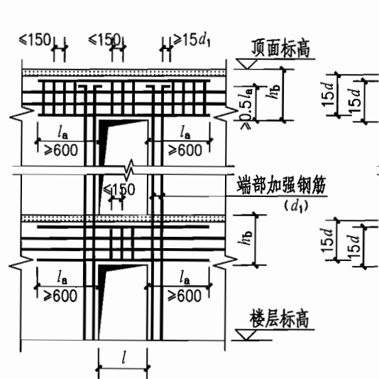
1 门洞连梁配筋示意
