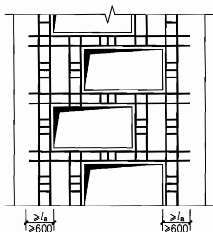
2 叠合错洞
