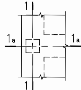
4 宽扁梁平面布置示意 (二)
