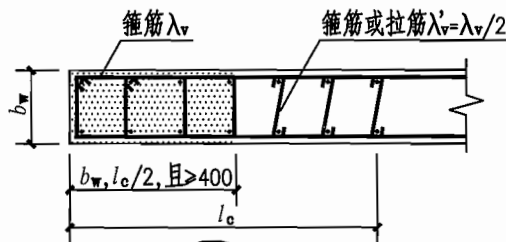
⑤ 暗柱
