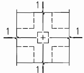
3 宽扁梁平面布置示意 (一)
