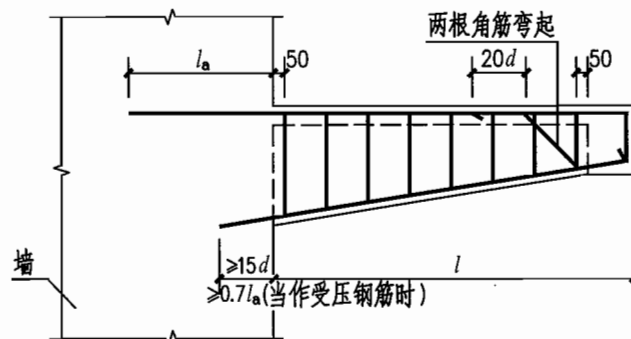
4 悬臂梁构造 (三)
