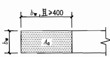
① 暗柱
