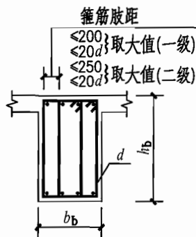
3 梁箍筋肢距要求
