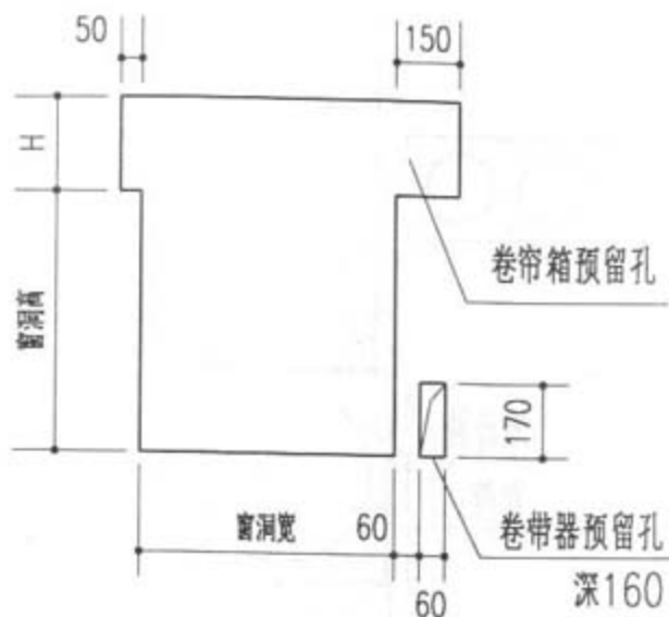
中装卷帘窗墙面预留孔
