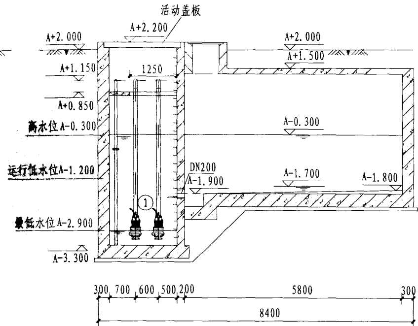
II-II 剖面图
