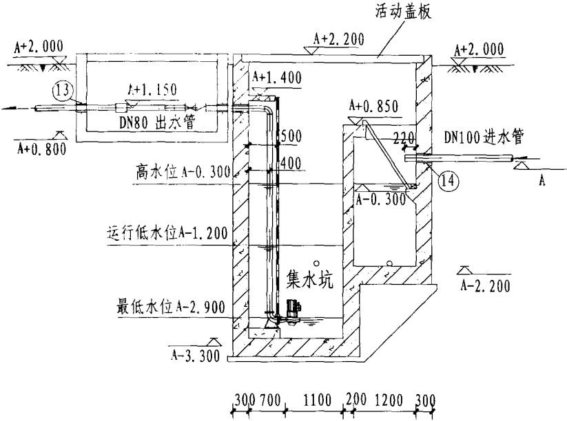
III-III 剖面图
