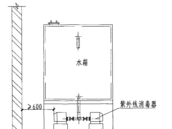
II-II 剖面图
