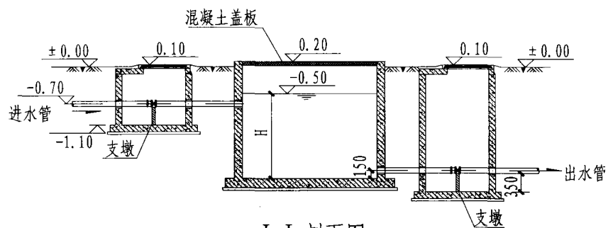
I-I 剖面图
