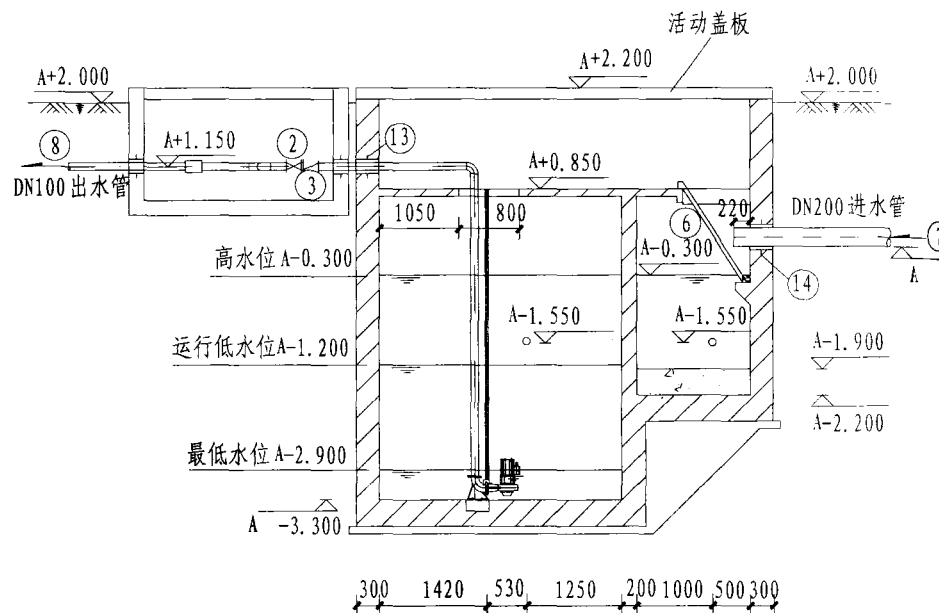
III-III 剖面图
