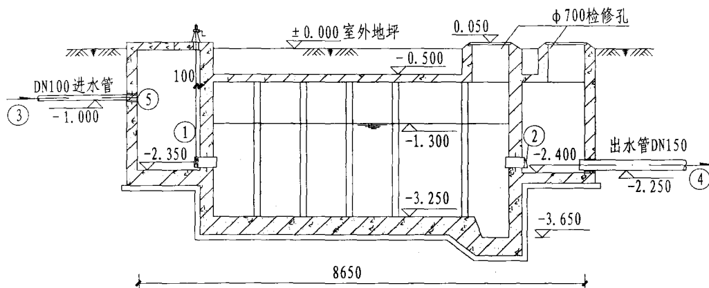
I-I 剖面图
