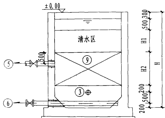
II-II 剖面图
