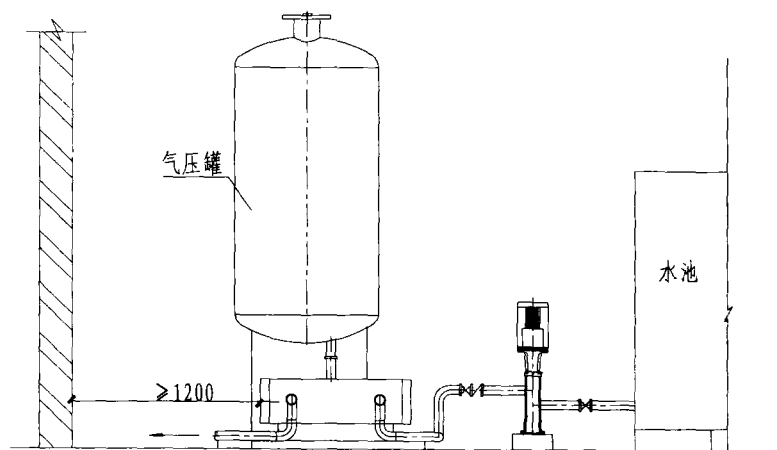
I-I 剖面图
