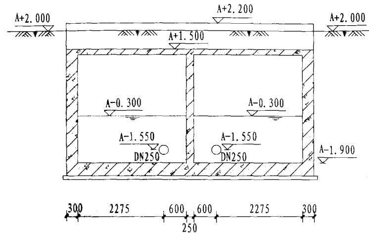
II-II 剖面图
