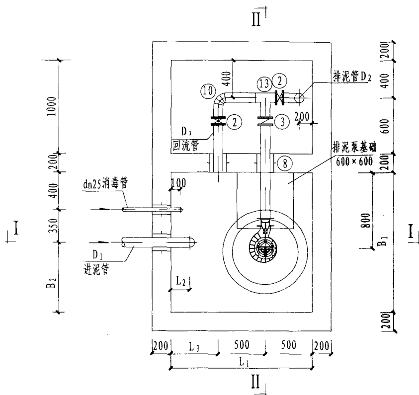
污泥消毒池平面图
