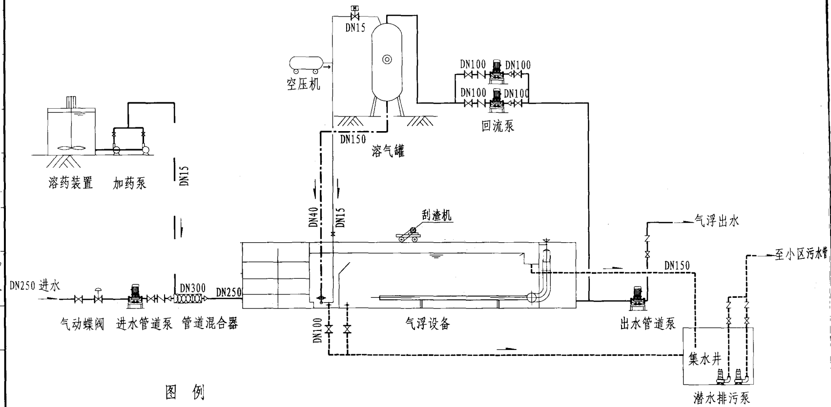
工艺流程图
