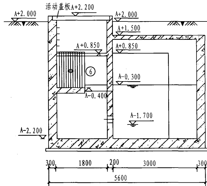
I-I 剖面图
