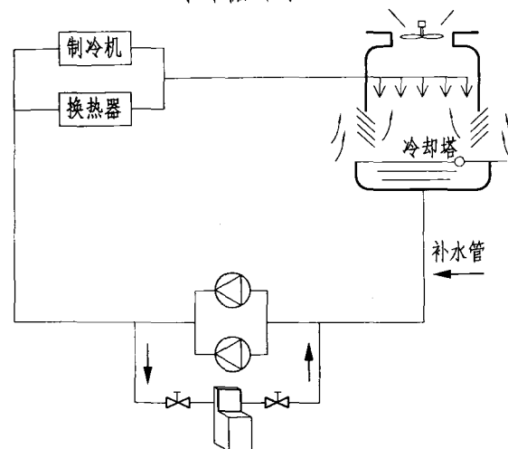
冷却循环水
