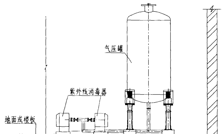
II-II 剖面图
