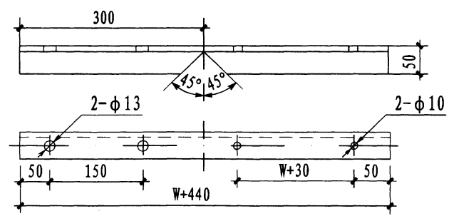
角钢支架
