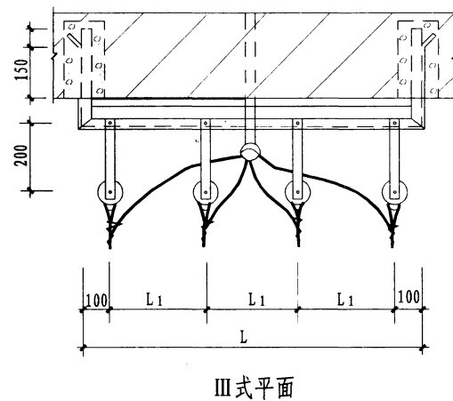
低压架空引入线安装做法(二)
