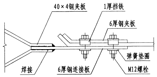
节点 1 立面
