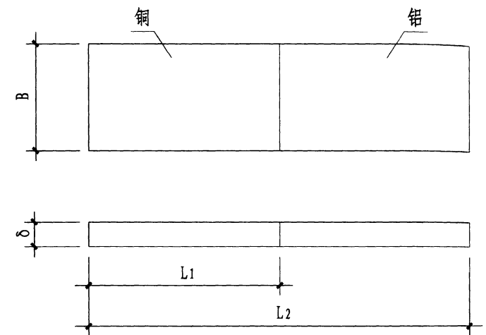
MG系列铜、铝过渡板
