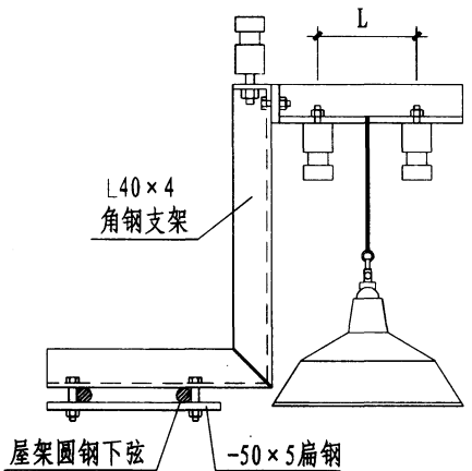
侧视(螺栓做法)
