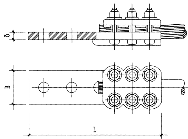
SL系列铝线夹
