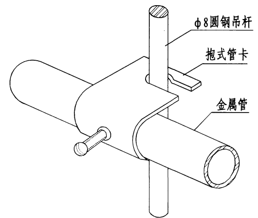
I 式 (独立设吊杆)
