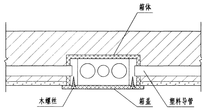
中途接线箱安装
