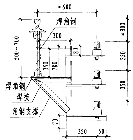
在钢梁上安装 I 式
