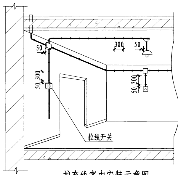
护套线室内安装示意图
