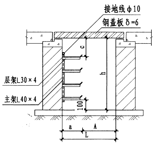
单侧支架电缆沟
