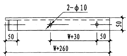
角钢支架
