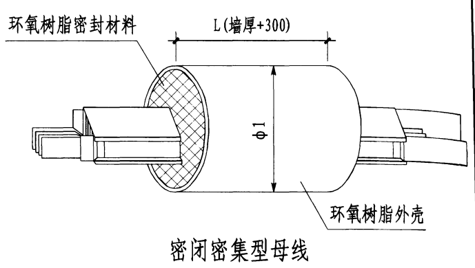
密闭密集型母线槽规格
