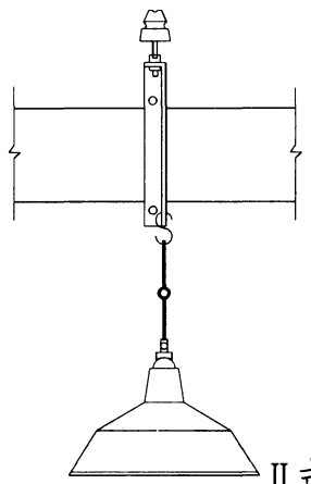
I 式支架(交叉) 正视
