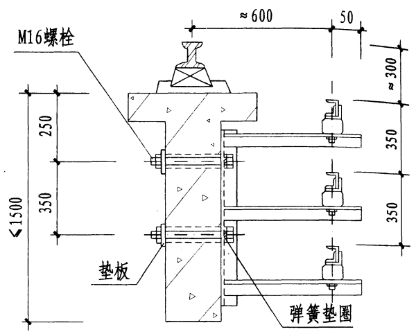
在钢筋混凝土梁上安装
