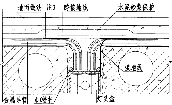
预制空心楼板灯头盒安装做法
