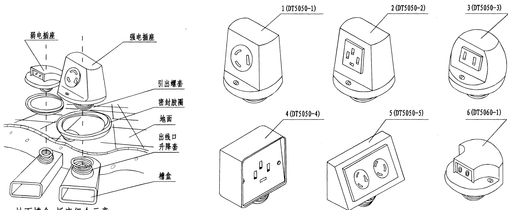
地面槽盒 插座组合示意
