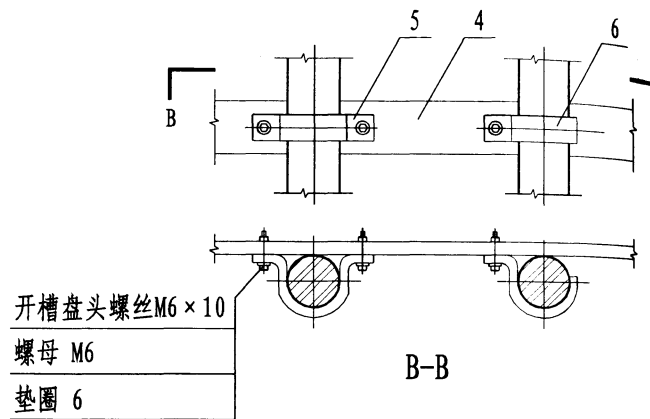
① 电缆沿墙敷设支架固定
