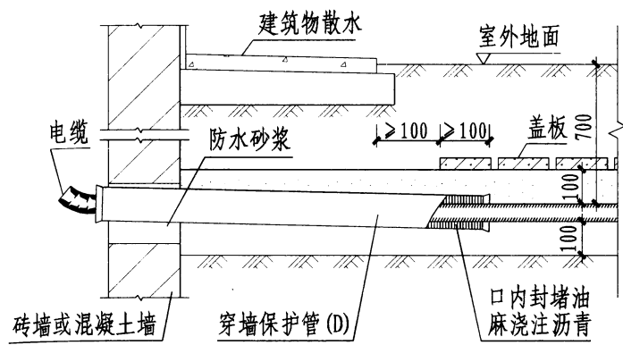
I 式剖面
