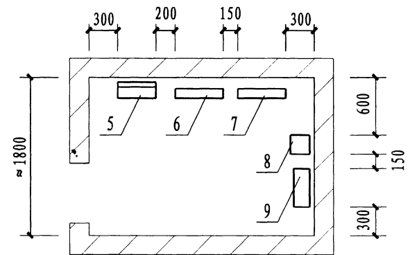
弱电竖井
