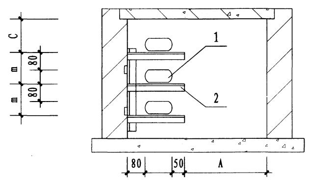
在电缆沟中安装
