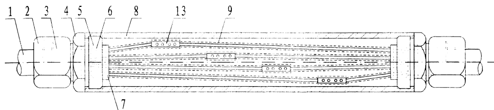
多芯电缆直通式中间连接器
