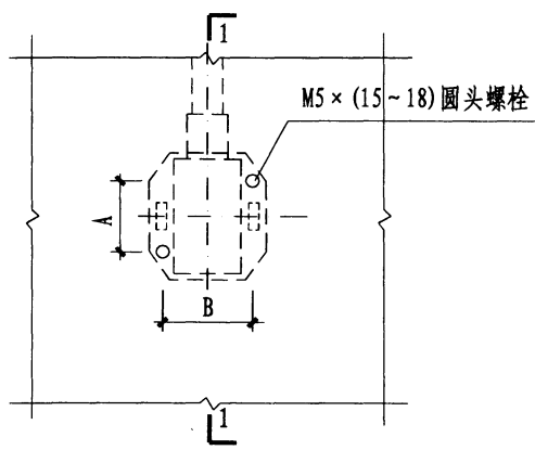
I型正视图
