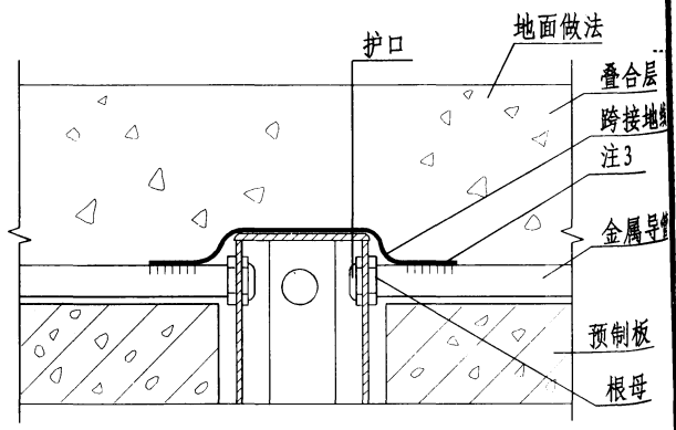
高桩灯头盒在预制板上安装做法
