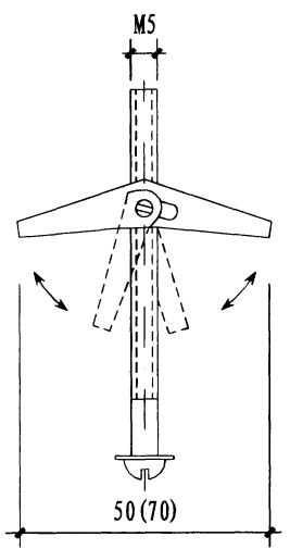
伞形螺栓
