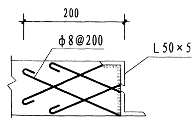
角钢埋件方案 II
