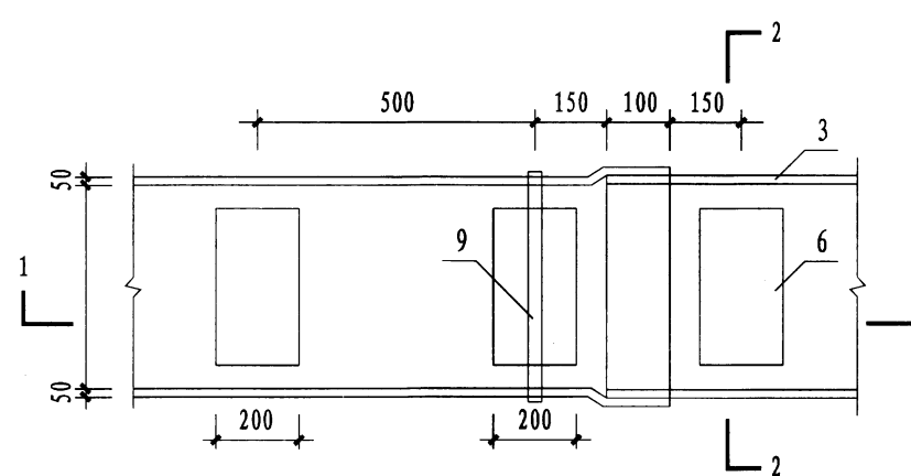
难燃封闭槽盒平面图
