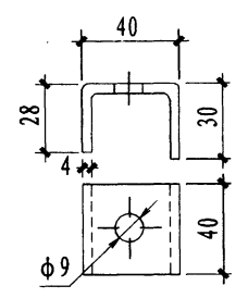
压板1
