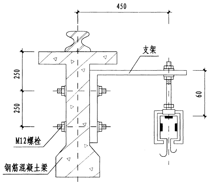
3号支架
