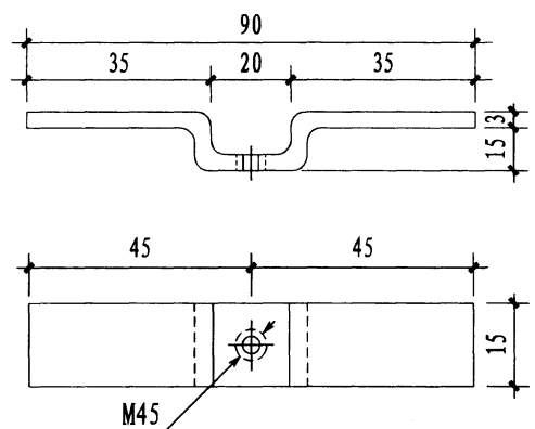
弓形铁板
