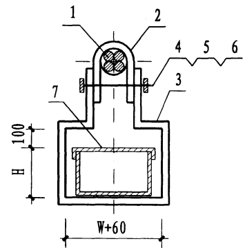
A-A 钢索吊槽盒示意图
