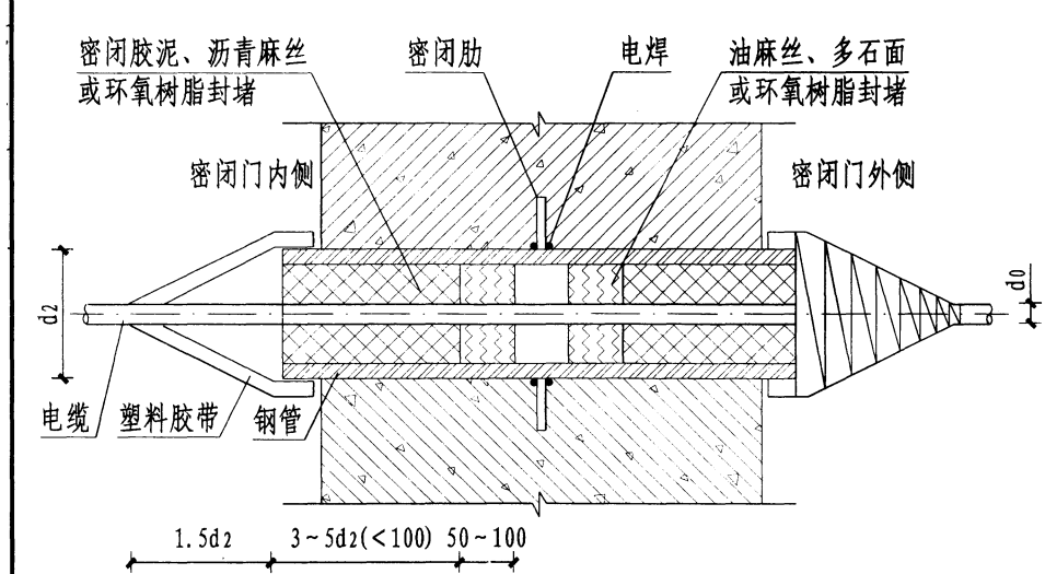
② 电缆穿密闭墙做法
