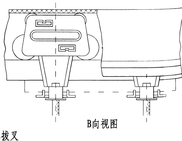
导管式安全滑触线安装示意图
