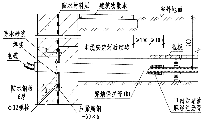
II 式剖面
