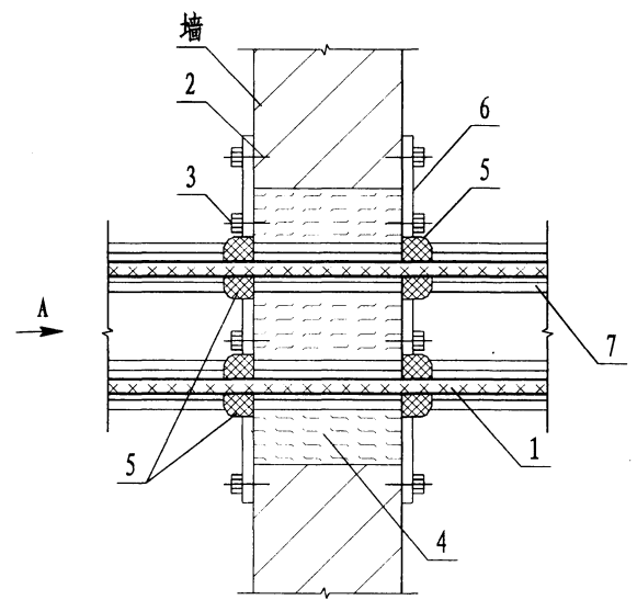
I 穿墙处密封示意图
