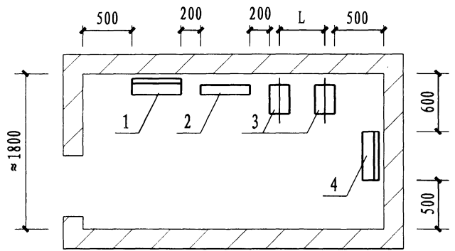
配电竖井
