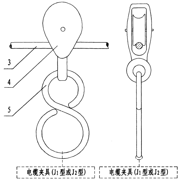
吊索上滑轮悬挂装置
