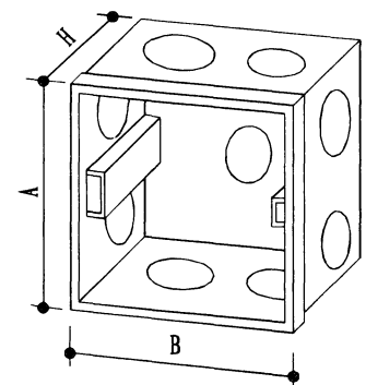
塑料盒 (86HS40、50、60)
