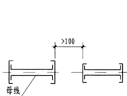
II 母线水平(平装)安装间距要求
