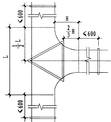
水平三通
