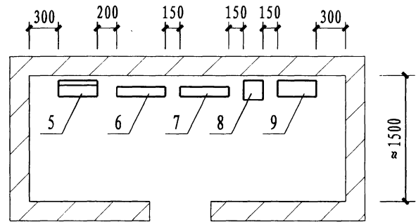
弱电竖井
