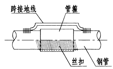
非镀锌金属导管丝扣连接
