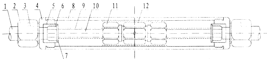
单芯电缆直通式中间连接器
