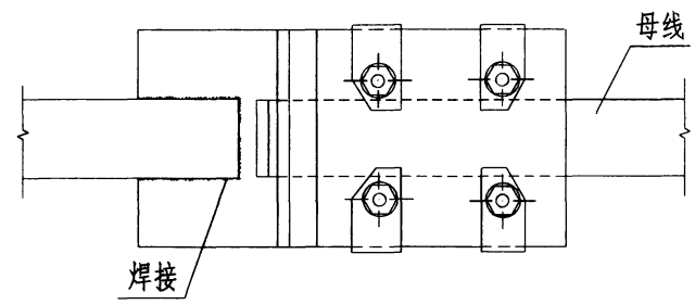
节点 1 平面
