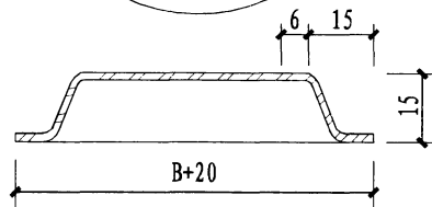
缩口盖板
