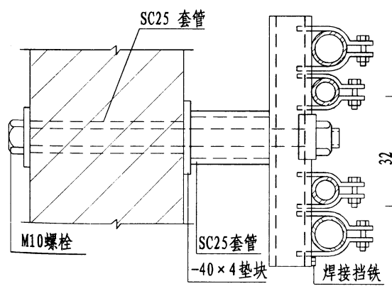
管卡槽垂直安装
