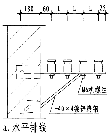
墙上扁钢支架安装做法
