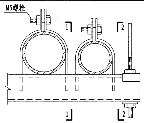
管卡槽水平安装
