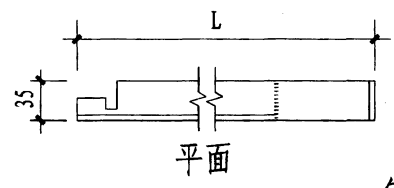
U型槽管卡
