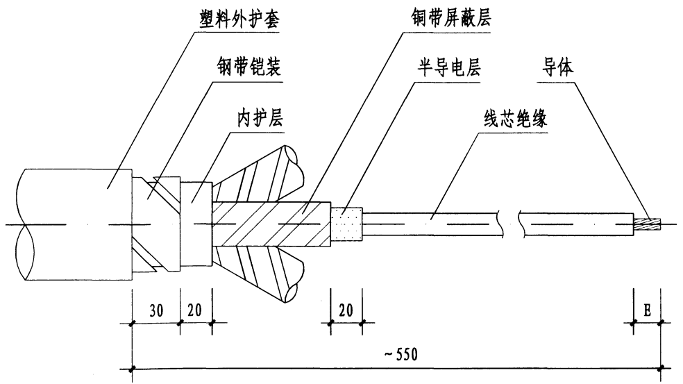
热缩型交联聚乙烯绝缘电缆终端头剥切尺寸
