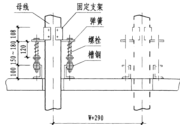
母线垂直安装(不带防火封堵)
