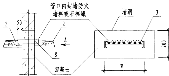
方案 IV A向
