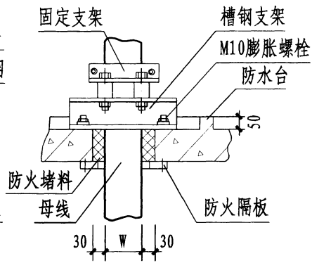
母线垂直安装(带防火封堵)
