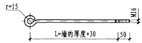
8号零件(二型)
