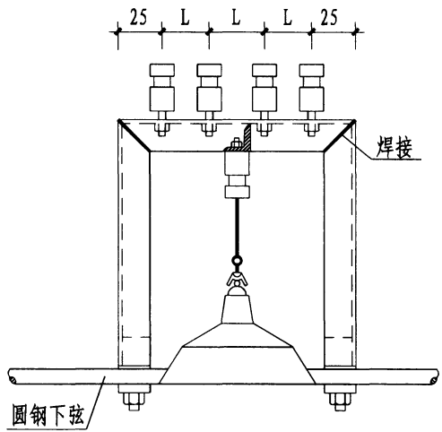
正视
