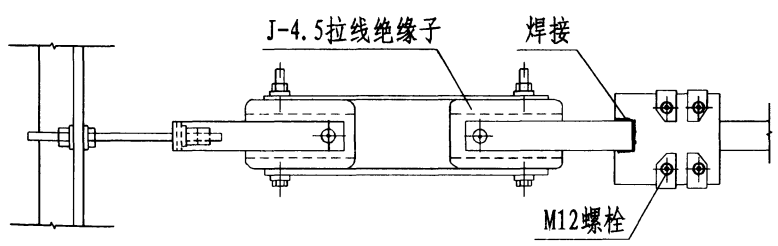
母线终端拉紧装置平面
