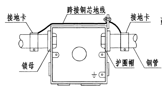
镀锌金属导管与金属盒连接
