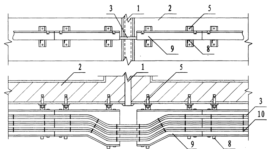
电缆在桥架内敷设
