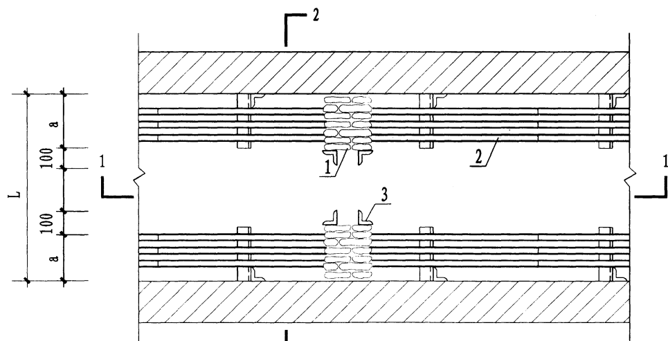
平面图
