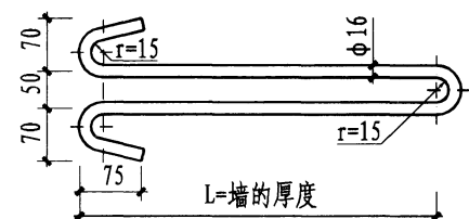
1号零件(一型)
