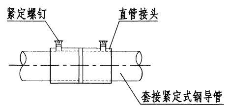
套接紧定式金属导管紧定螺钉连接
