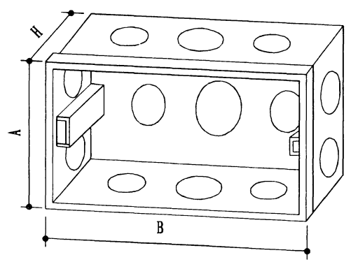
塑料盒 (146HS50、60)
