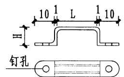
双线卡 (金属)
