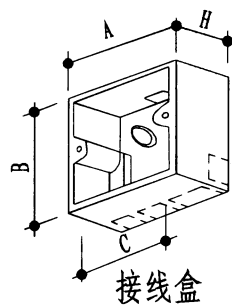
槽盒与明装接线盒安装做法(一)
