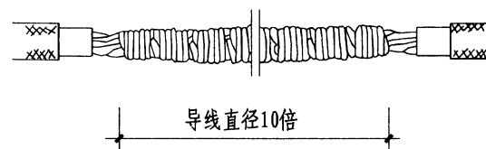
直线连接(二式)
