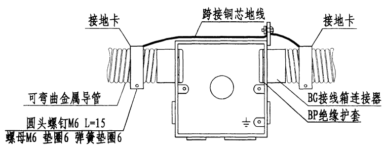
可弯曲金属导管与金属盒连接
