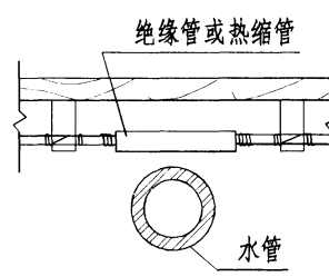
导线与水管交叉做法
