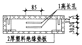
1-1剖视
