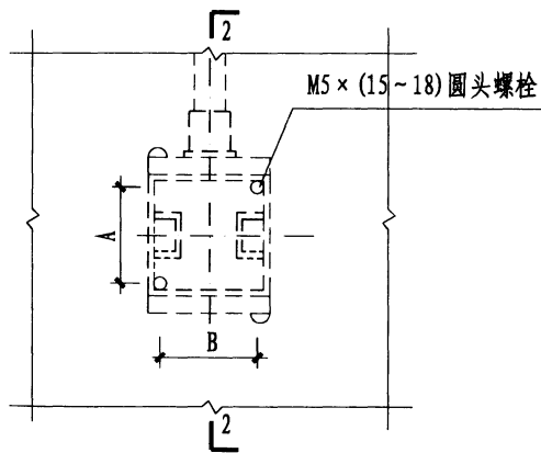
II型正视图
