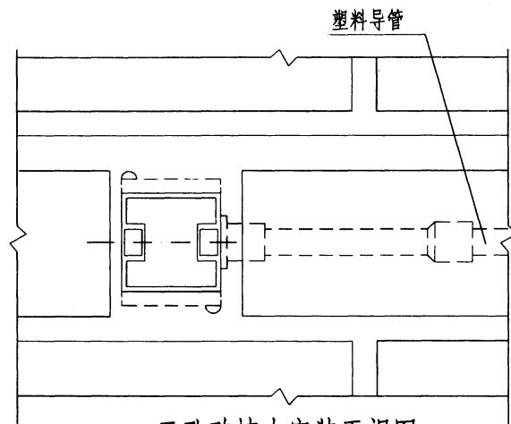
三孔砖墙内安装正视图
