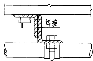
角钢支架连接做法
