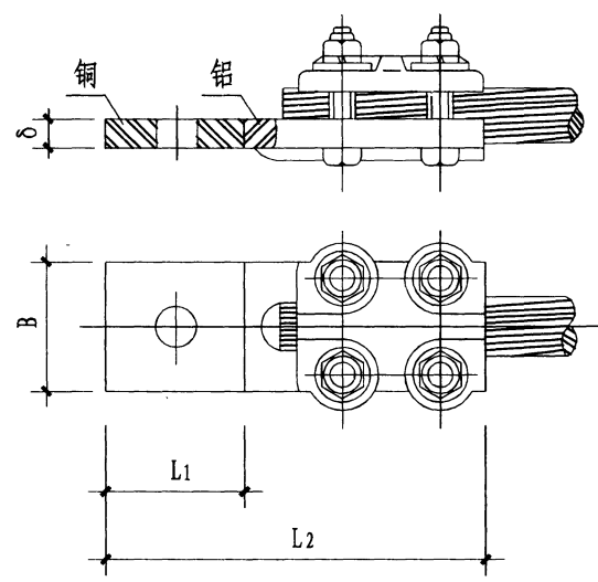
单孔型
