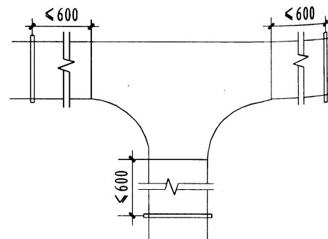
垂直三通
