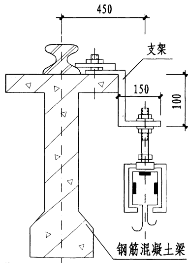
2号支架
