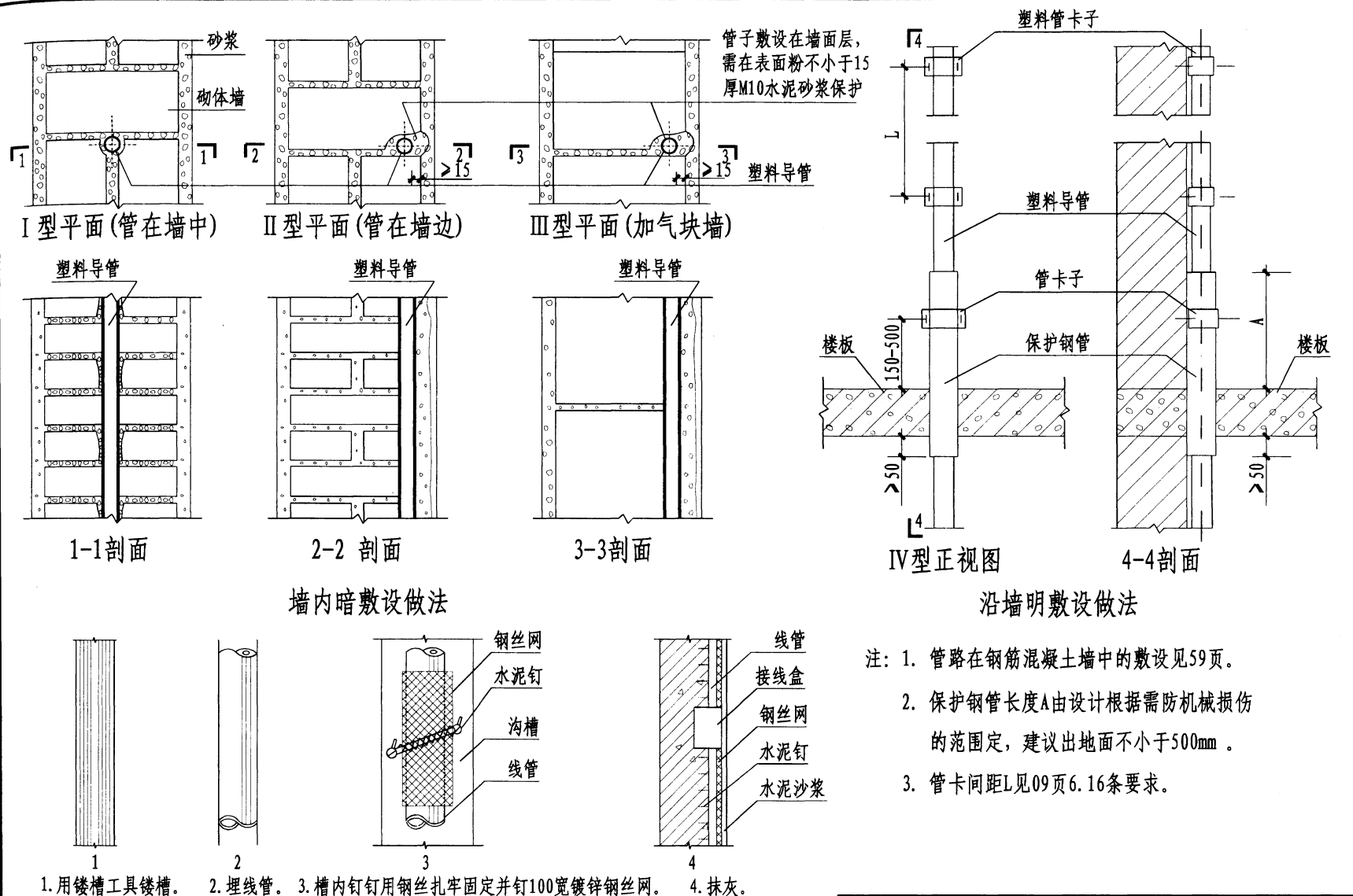
改建工程 II、III型做法工序
