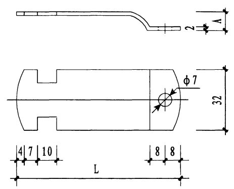
U型槽管卡
