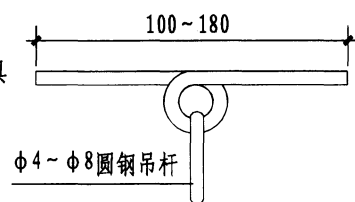
灯具及吊杆
