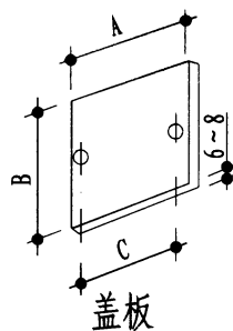
槽盒与明装接线盒安装做法(二)
