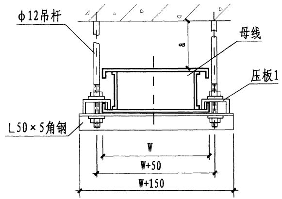
母线吊装 III
