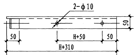
角钢支架
