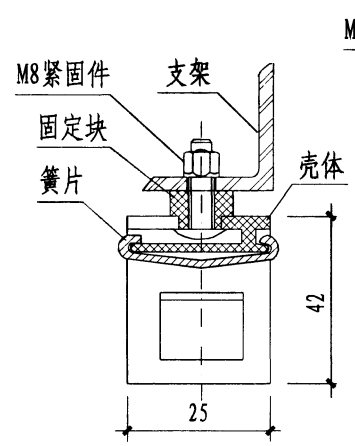
I 型吊挂夹
