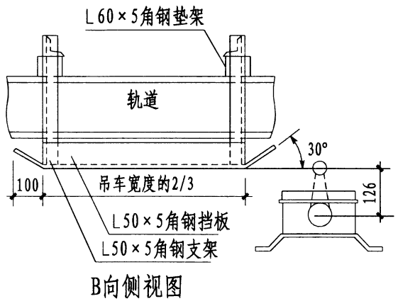
悬挂梁式吊车限位开关操作挡板安装
