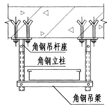
角钢吊架式
