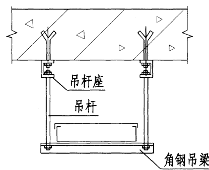
圆钢吊架式
