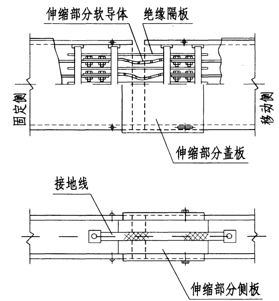
母线伸缩节
