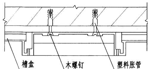
I - I 剖面
