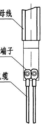
母线与电缆连接
