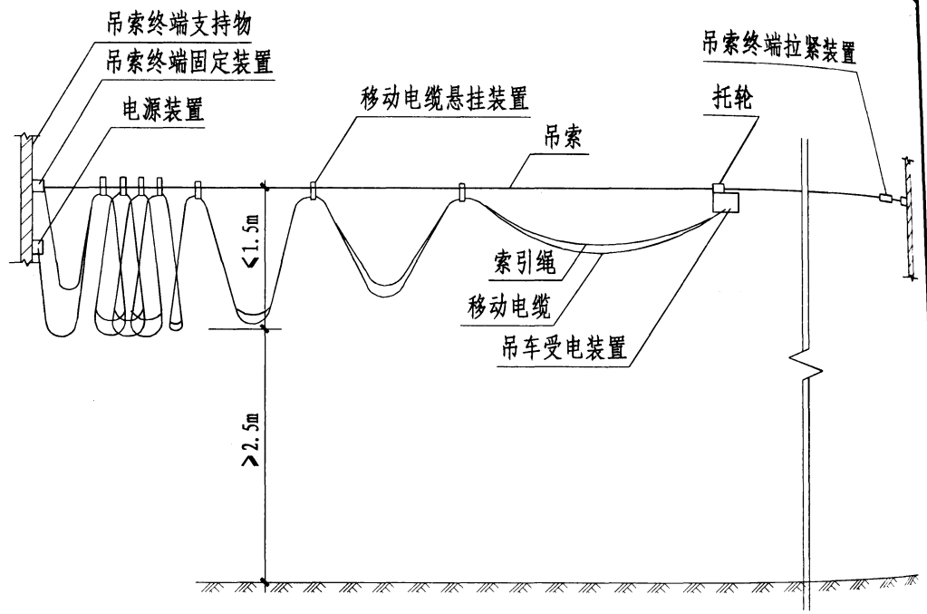
吊索悬挂移动电缆示意图
