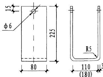
MC型母线立柱式安装
