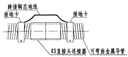
可弯曲金属导管连接
