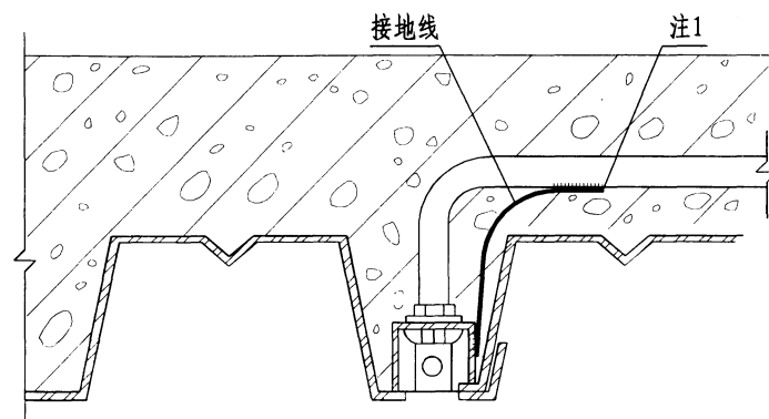
无吊顶做法
