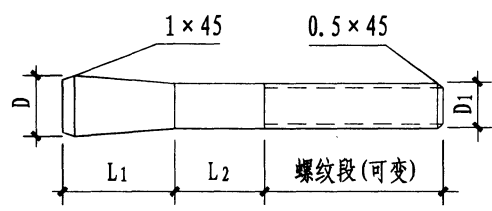
螺栓
