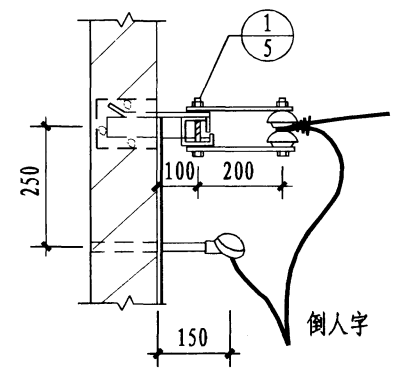
I 式侧视
