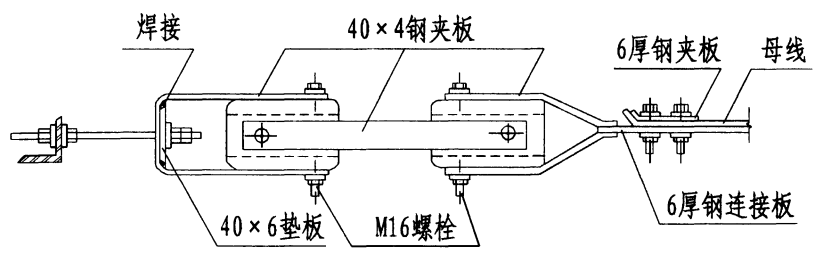
母线终端拉紧装置立面
