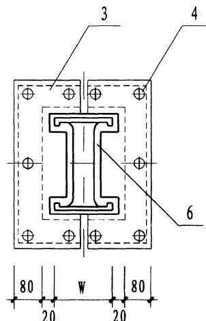
A向
