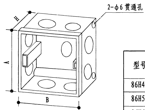
塑料盒 (86HSG50、60)
