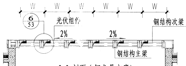
2-2 剖面 (钢龙骨方案)
