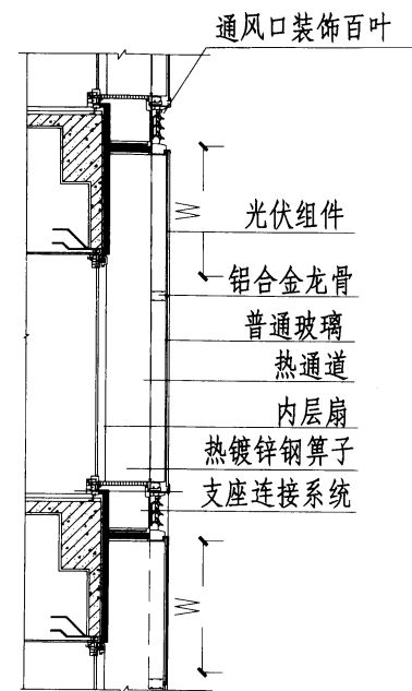
1-1 剖面图
