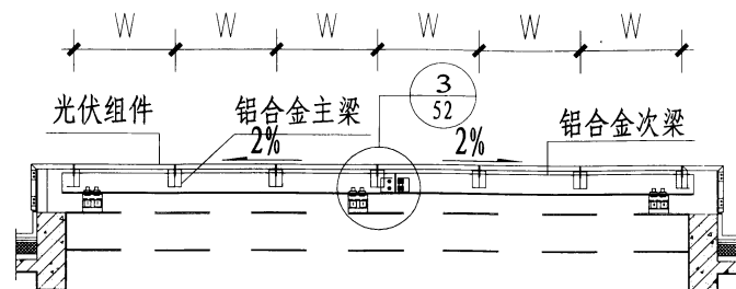
2-2 剖面 (铝龙骨方案)
