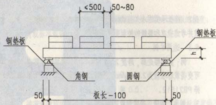
加载示意图
