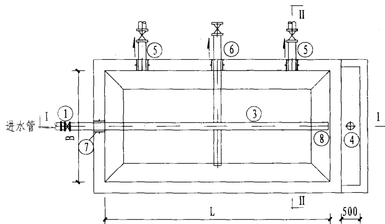
水解池平面图
