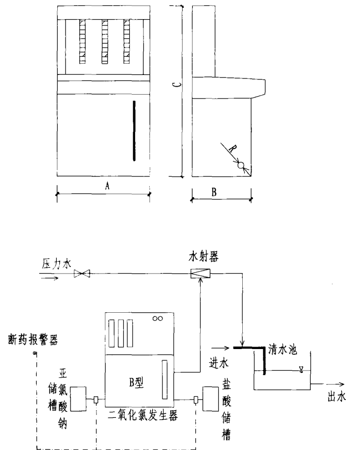
负压式二氧化氯发生器外型及投加原理
