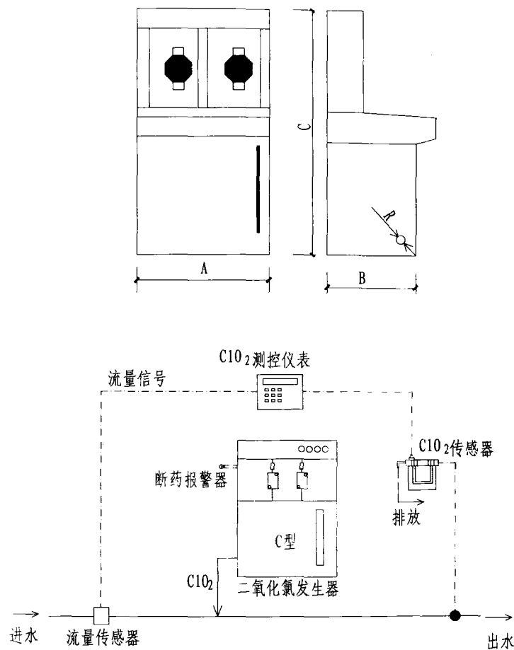
正压式二氧化氯发生器外型及投加原理
