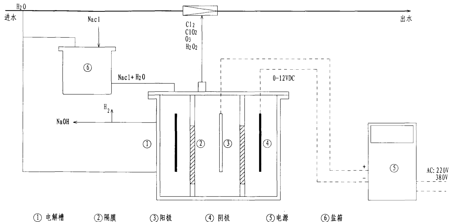
电解法二氧化氯投加量
