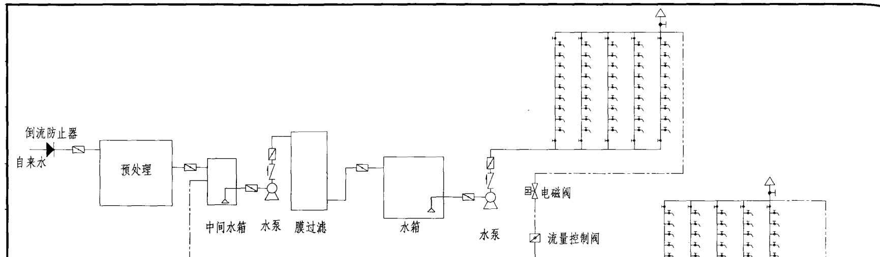
变频调速泵供水系统示意图
