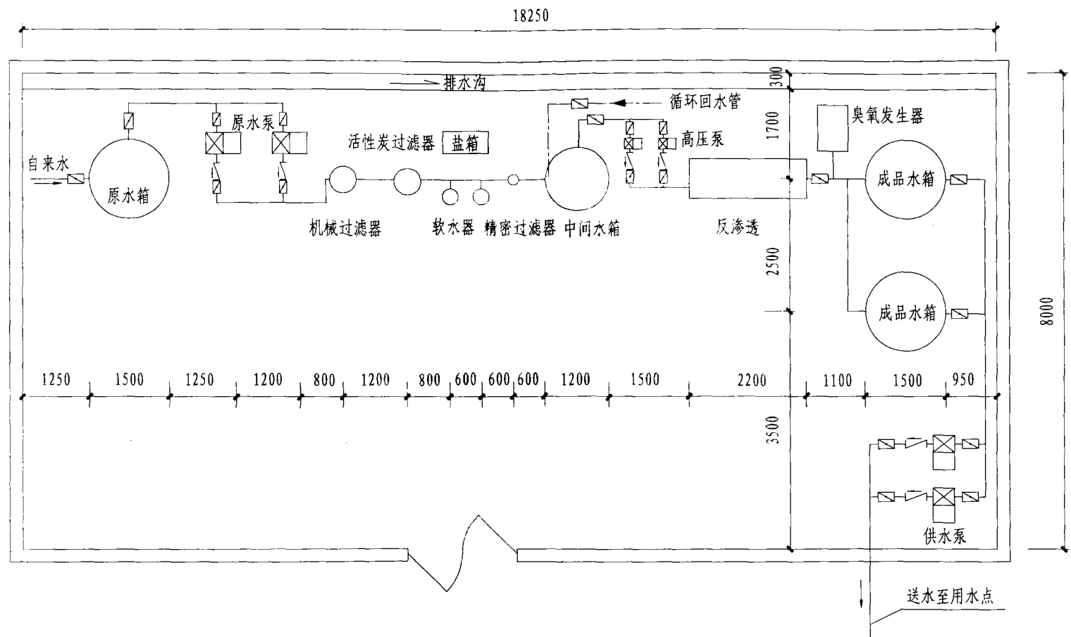
平面布置图
