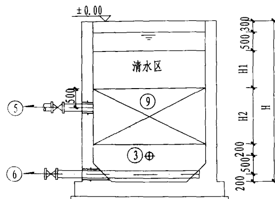
II-II 剖面图
