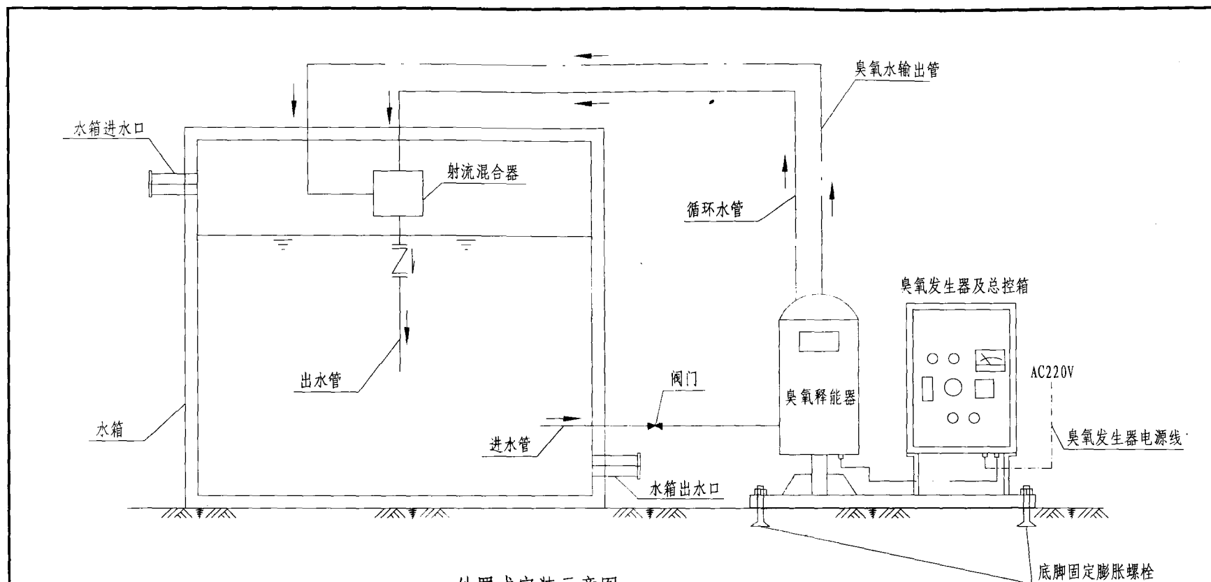
外置式安装示意图
