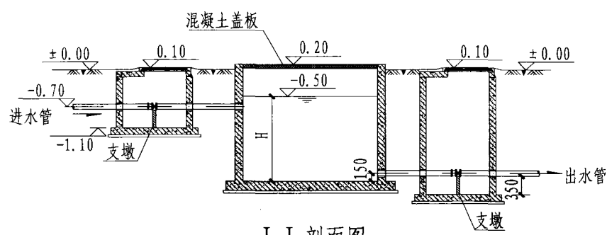
I-I 剖面图
