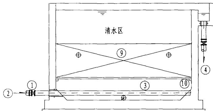
I-I 剖面图
