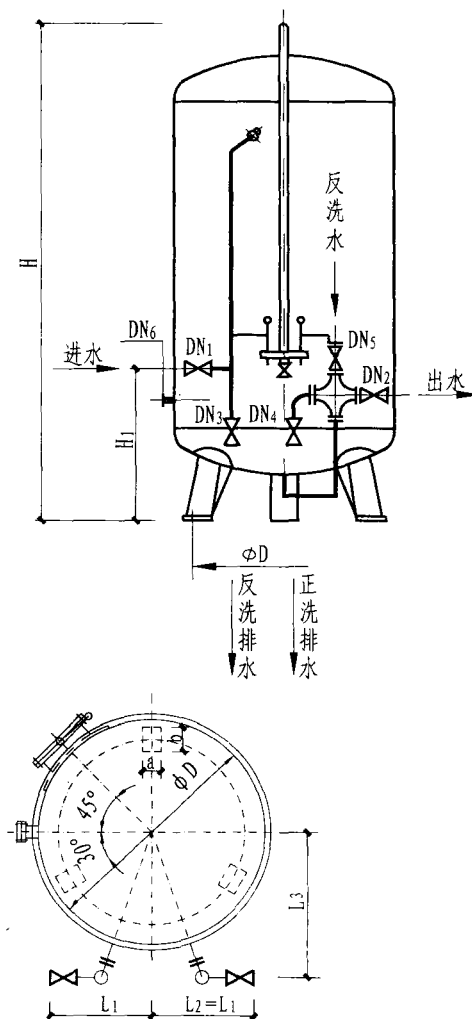
活性炭过滤器
