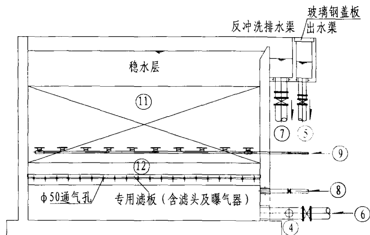
I-I 剖面图
