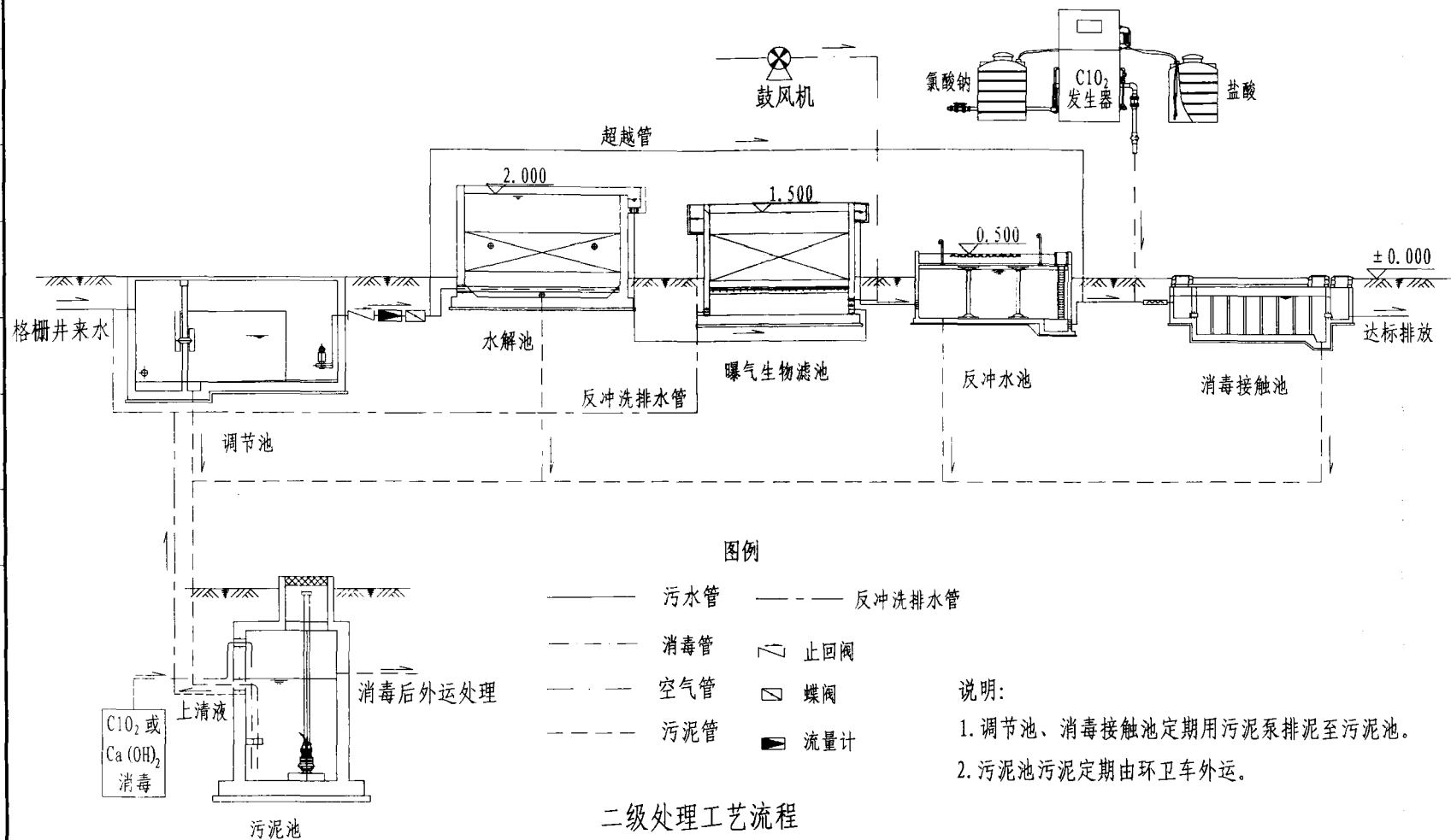
二级处理工艺流程 (二)
