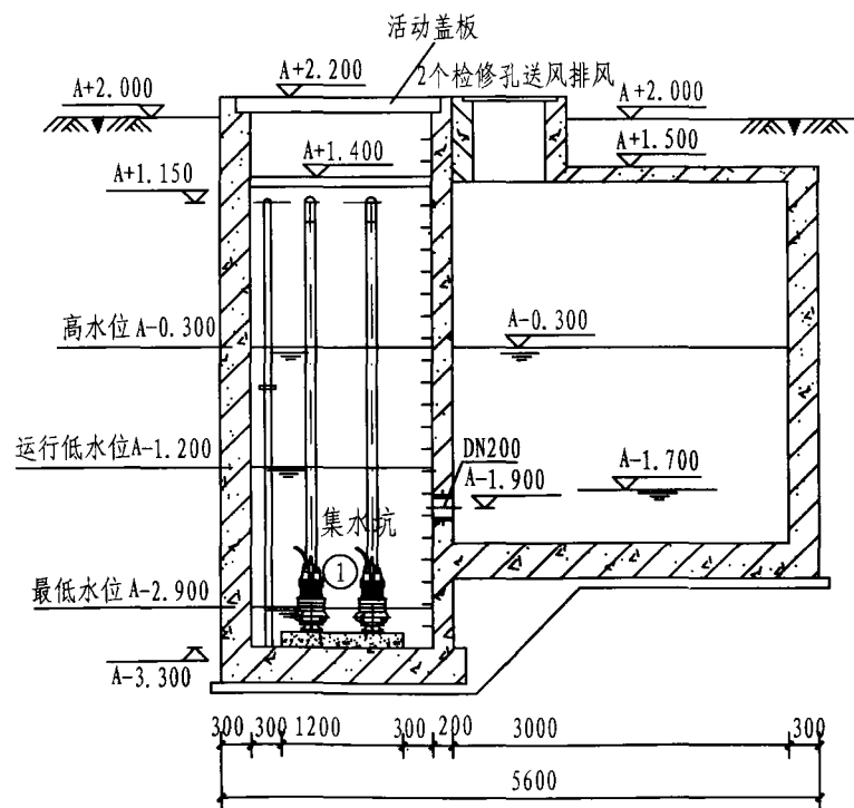
II-II 剖面图
