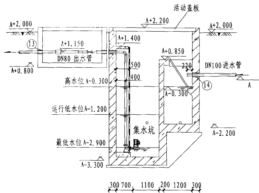
III-III 剖面图
