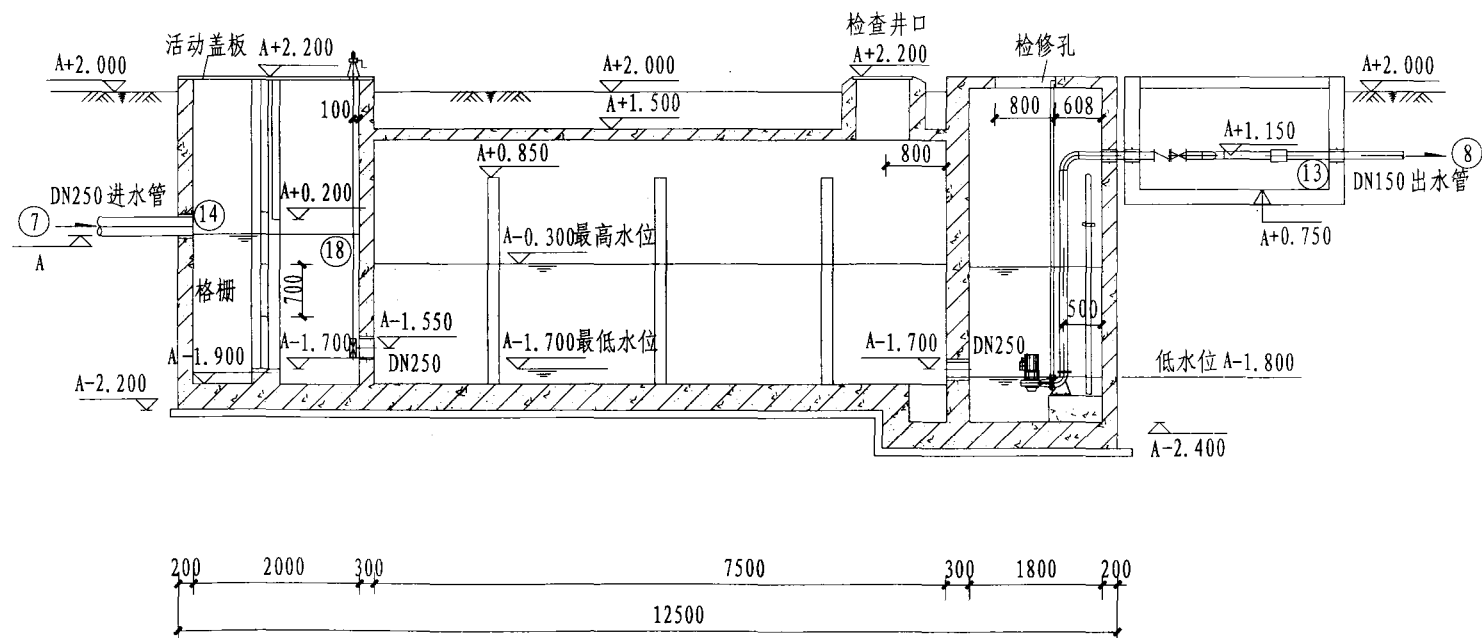
I-I 剖面图
