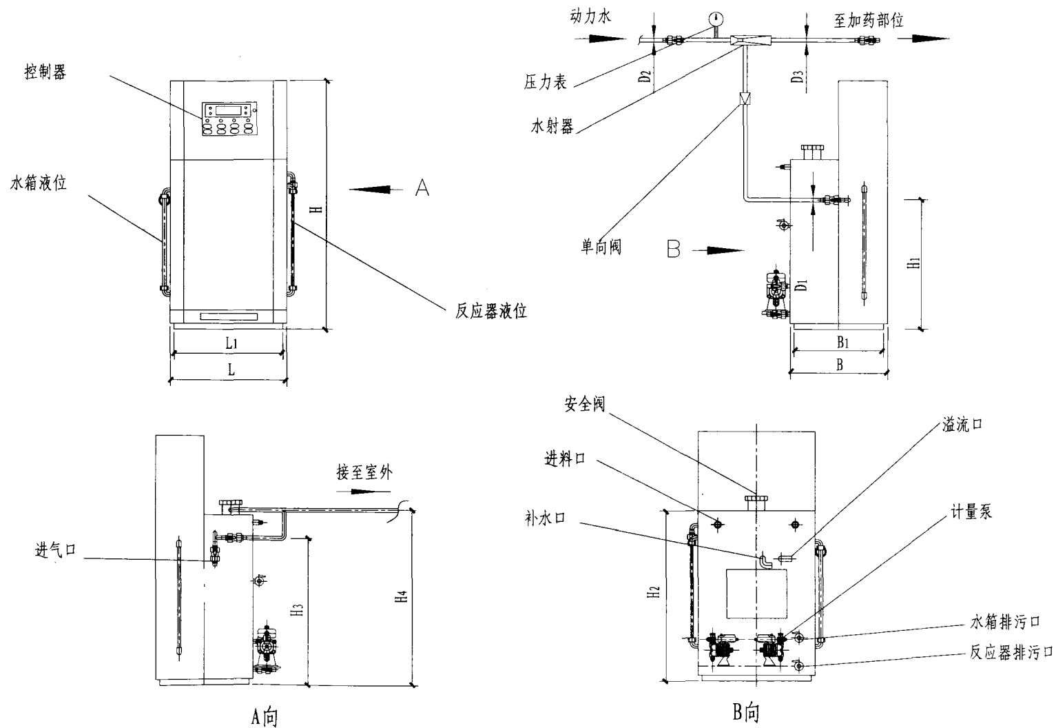
化学法二氧化氯发生器安装图 (三)
