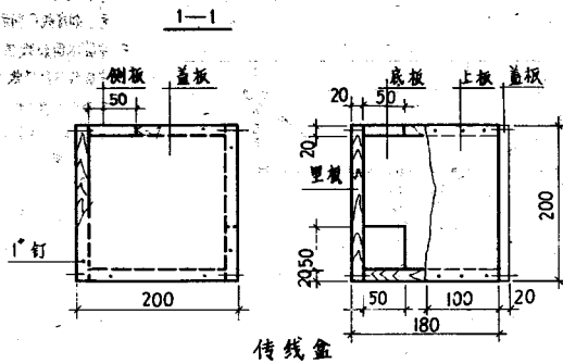
传线盒安装
