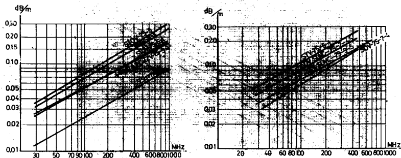
同轴电缆的衰减—频率特性曲线
