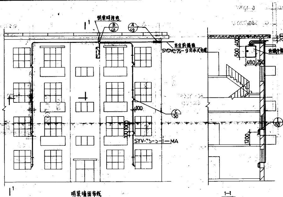
明装墙面布线
