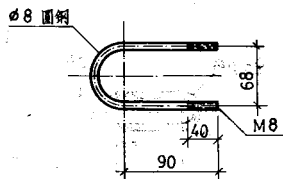
1 U形螺栓
