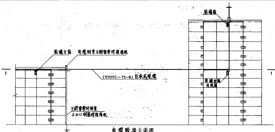
电缆跨接立面图
