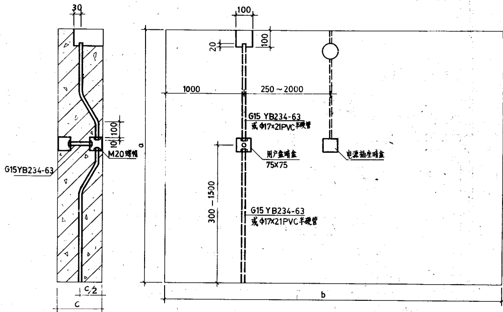
大板墙体预埋管方案I
