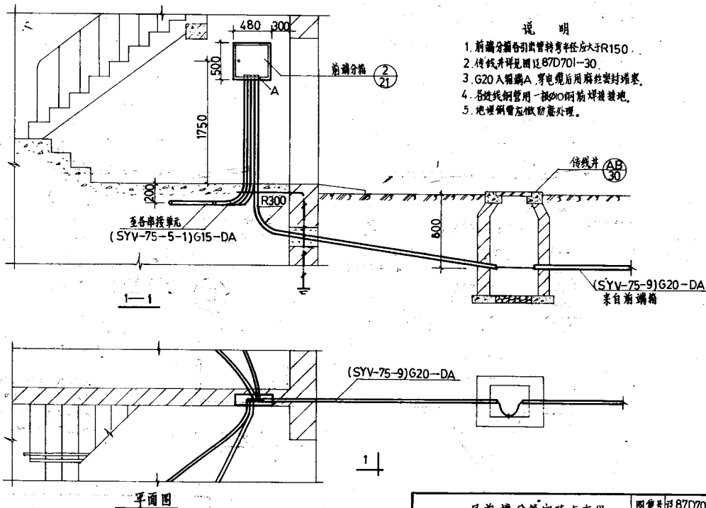
一层前端口箱安装与布线
