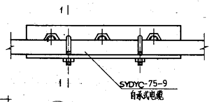
(3) 电缆固定
