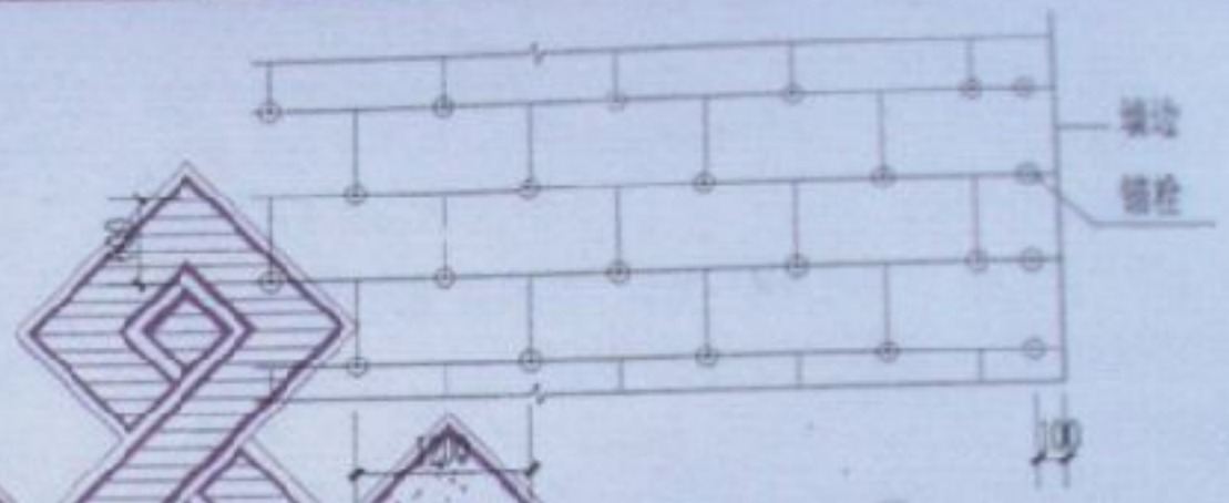
② EPS板排列及锚栓固定示意图
