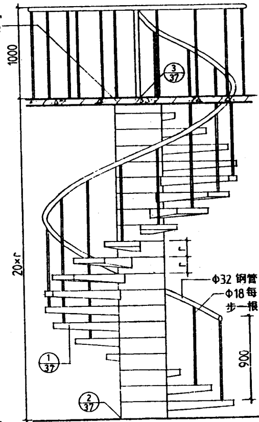
B 型立面
