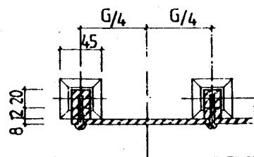
垫圈详图
