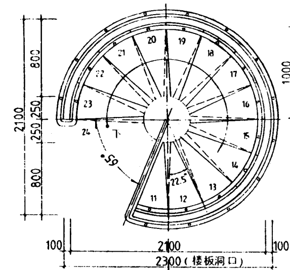
C型 2-2 平面
