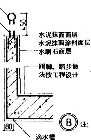
① 水泥抹面面层 ② 水泥抹面涂料面层 ③ 水刷石面层
