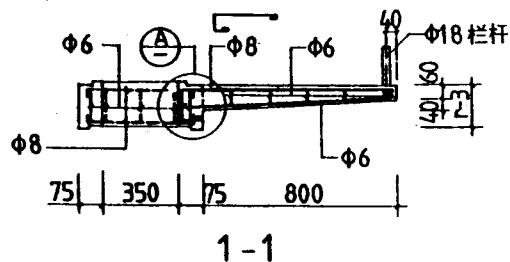
① 预制踏步板详图
