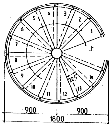
〔型 1—1 平面〕
