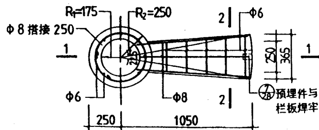
① 预制踏步板详图
