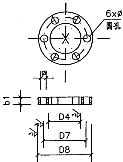
⑦ 法兰盘
