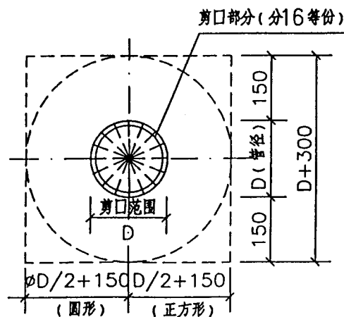
圆(方)形附加层做法
