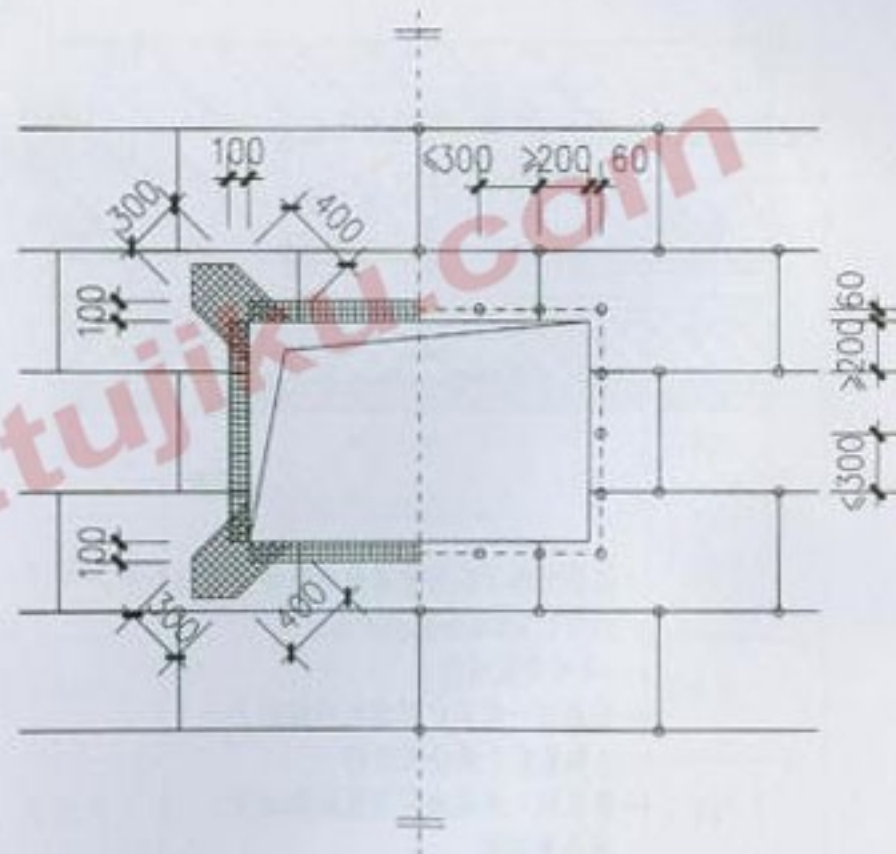
门窗洞口附加网格布及固定件布置
