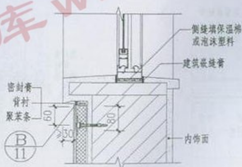
④ 窗居中，有窗套
