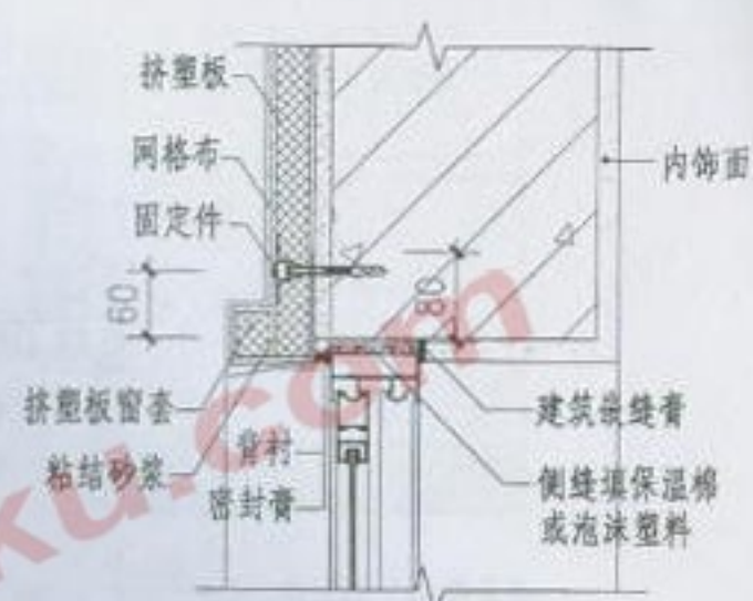
⑤ 窗居外侧，有窗套
