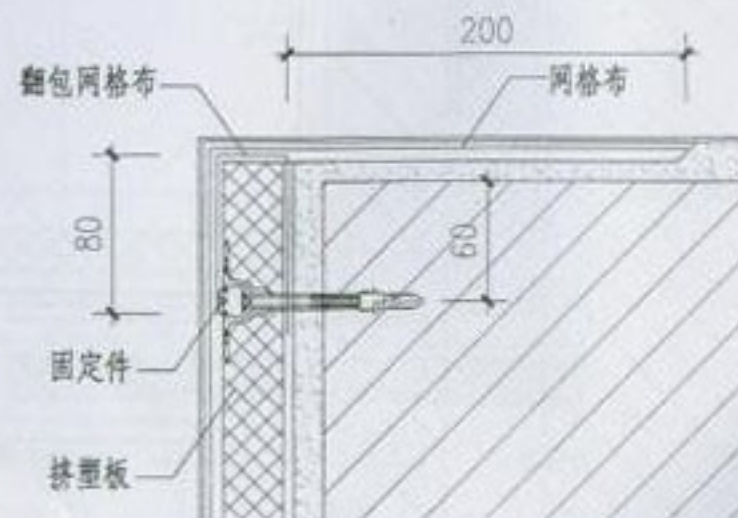
④ 保温墙体与不保温墙体连接详图
