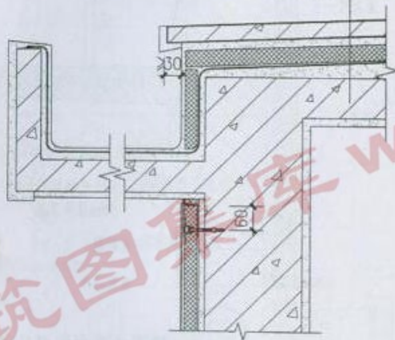
① 倒置式屋面保温构造
