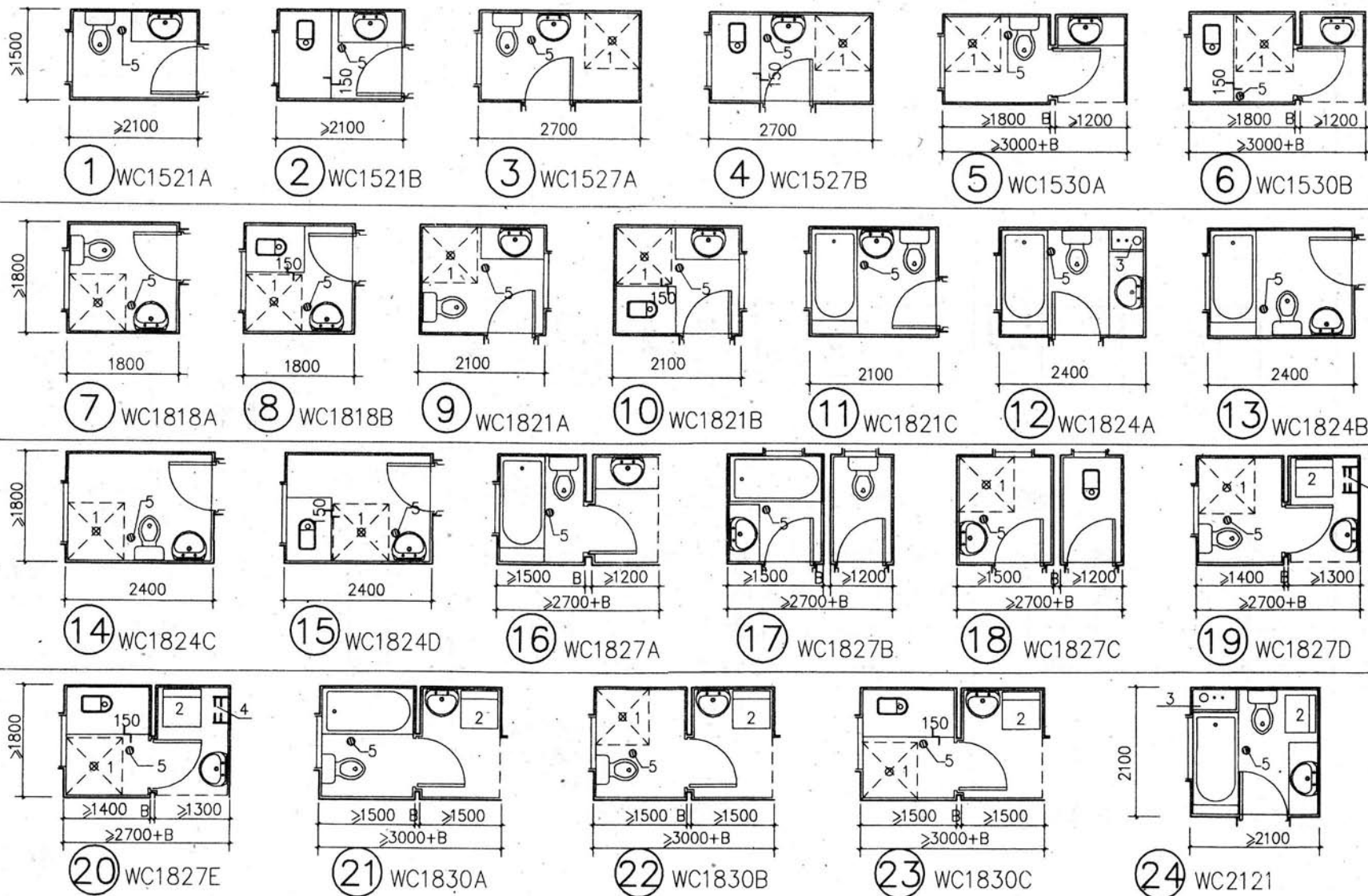
卫生间平面示意图
