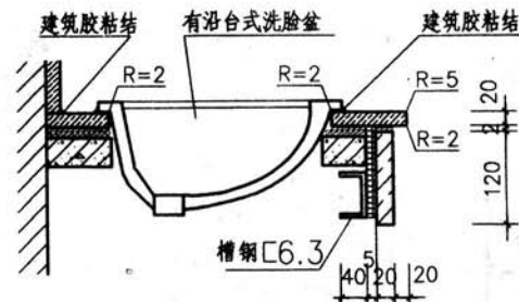
2-2 用于有沿台式洗脸盆
