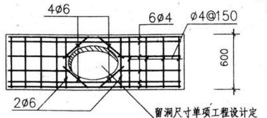
衬板配筋
