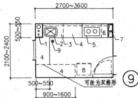
厨房平面示意图
