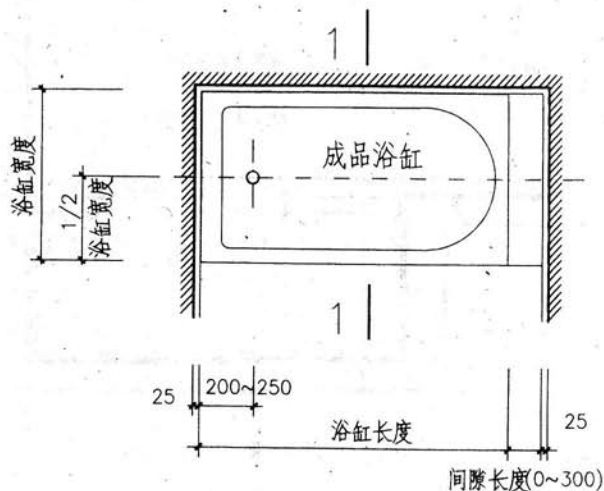
浴缸平面
