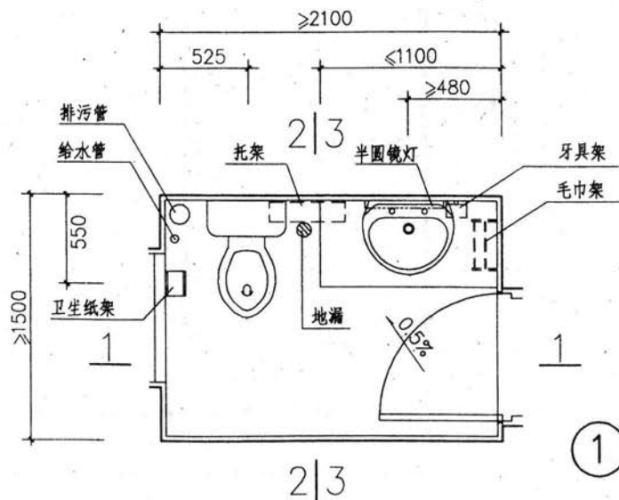
卫生间平面 (WC1521A)
