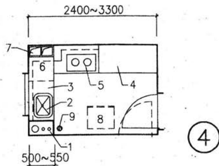
L形布置
