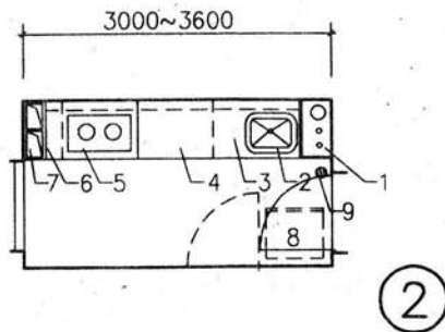
单排形布置
