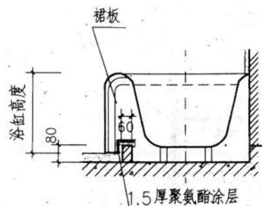
1-1 用于带裙板式浴盆
