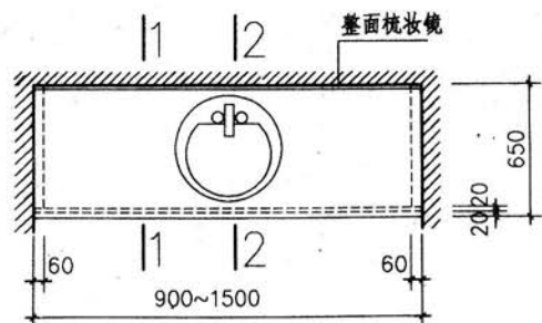
洗脸台平面、立面
