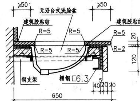
2-2 用于无沿台式洗脸盆
