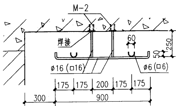
晒衣架 ①方钢 ①a圆钢
