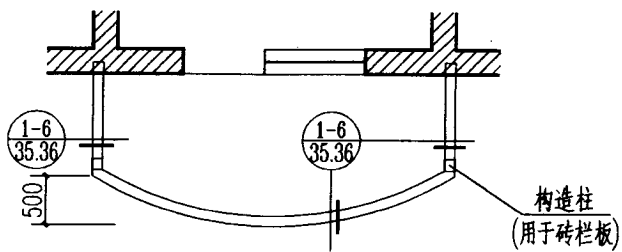
⑦号阳台平面
