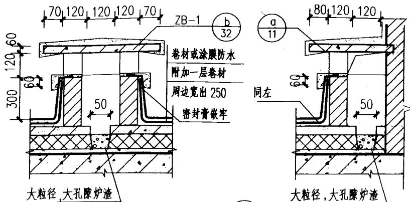
⑦ 边排汽管
