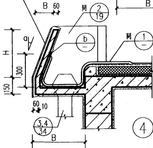
④ 带斜板天沟 (二)
