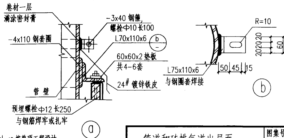
管道和砖排气道出屋面
