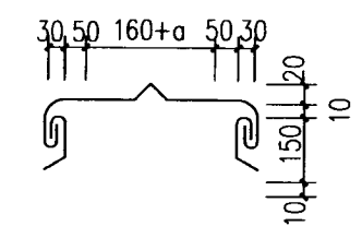
(b) 24# 镀锌铁皮
