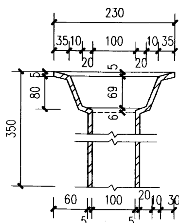
(d) 铸铁承水管
