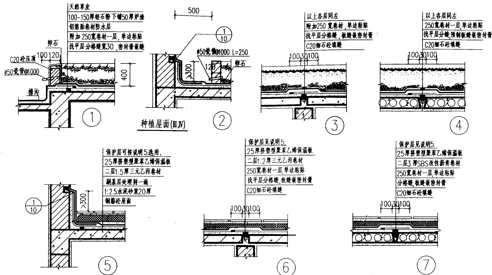
倒置式屋面(I, II)
