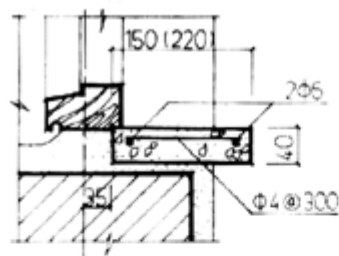
水泥窗台板
