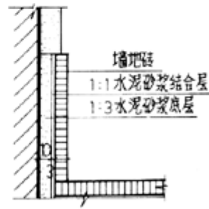
墙地砖踢脚
