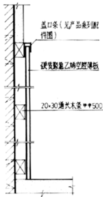
② 硬质聚氯乙烯 空腔薄板墙裙 1500高
