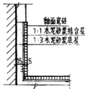
糙面瓷砖踢脚
