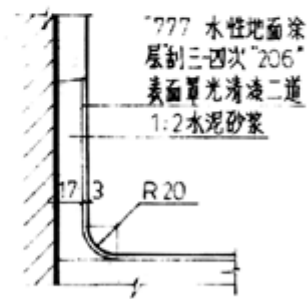
涂料水泥踢脚
