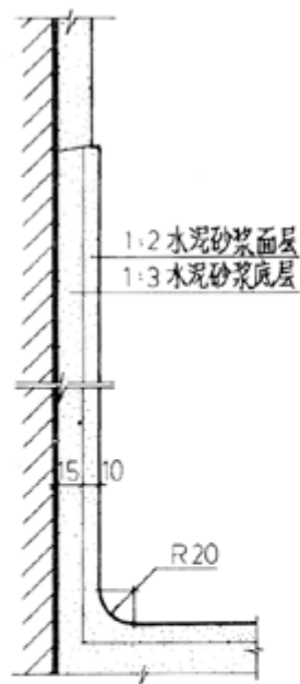
① 水泥墙裙 1500高
