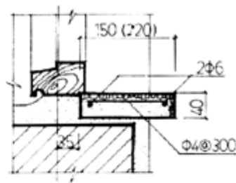
水磨石窗台板
