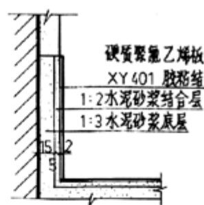
硬质聚氨酯板踢脚
