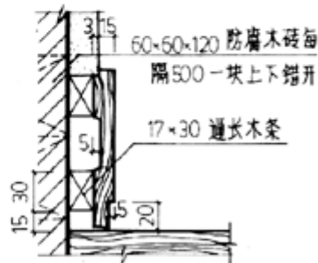
木踢脚
