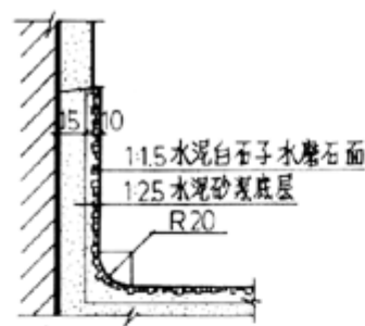
水磨石踢脚
