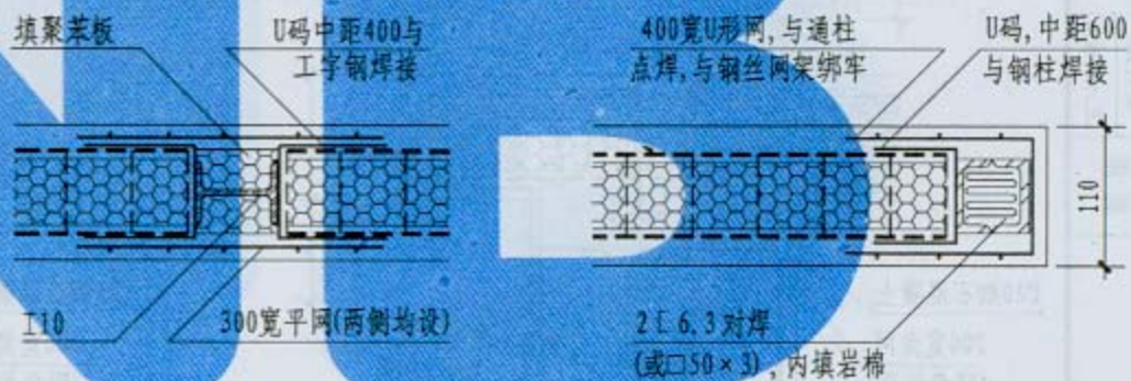
5 板墙加劲柱构造(三)
