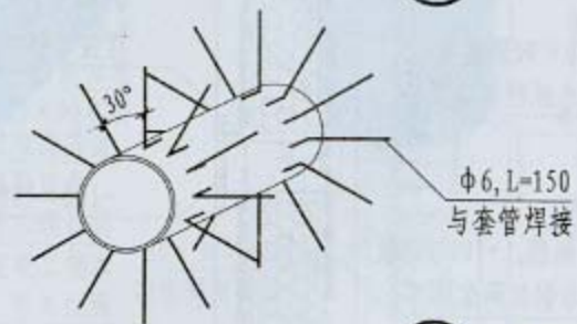
Ⓐ 穿墙套管
