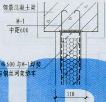
② 板墙与混凝土梁连接构造(二)
