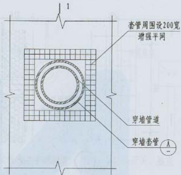
① 管道穿墙构造
