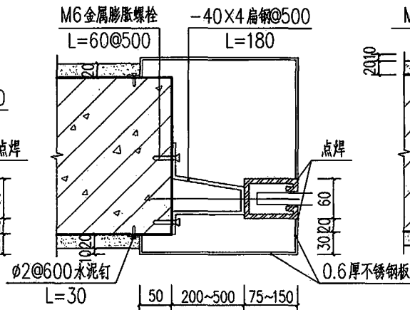
1a 不锈钢板装修
