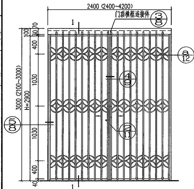
LZM201a-2430立面 (关闭时)
