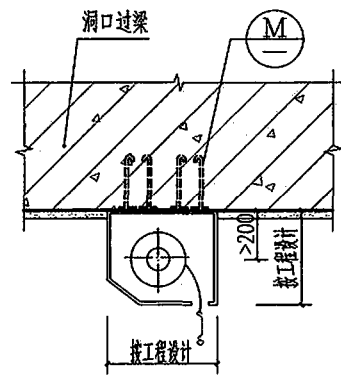
⑥ 墙体中间安装
