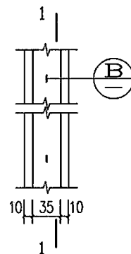
④ 固定边框闭门舌构造
