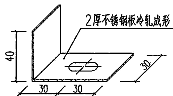
⑤ 门底横框固定角码
