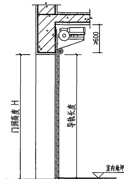
1-1剖面图
