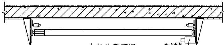
电机处平面图
