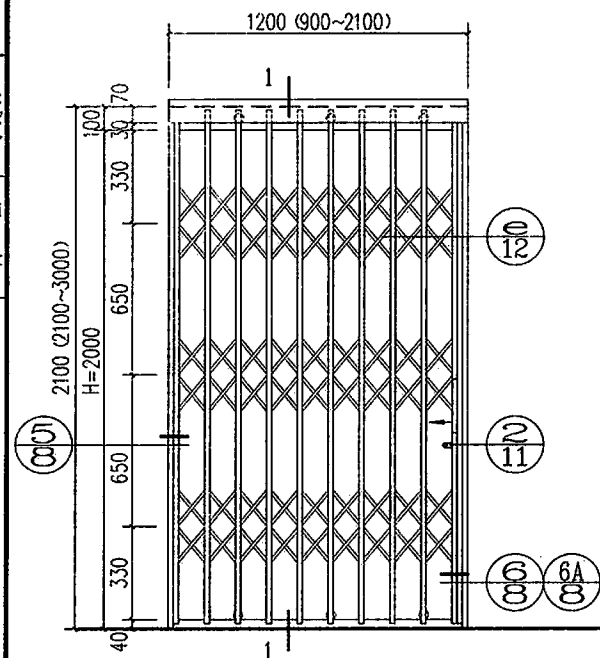
LZM101e-1221立面 (关闭时)
