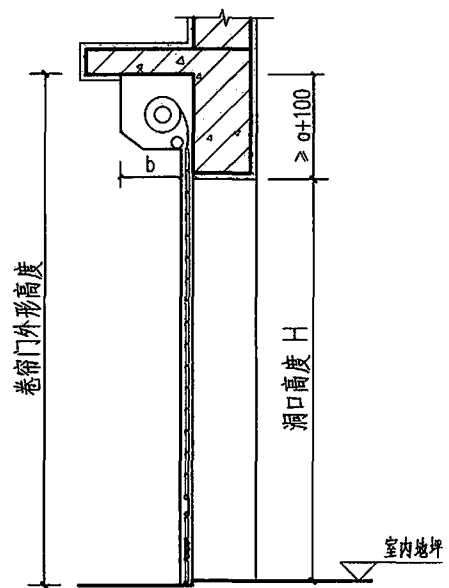
1-1剖面图
