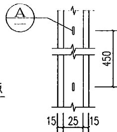
③ 活动边框闭门孔构造
