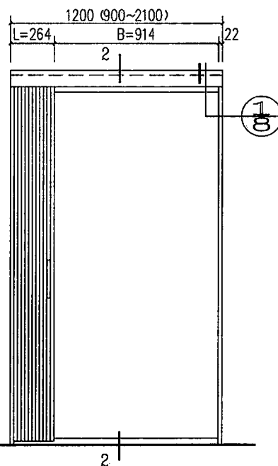
LZM101e-1221立面 (开启时)
