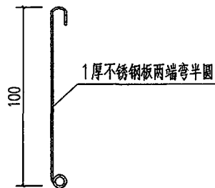
① 门顶装饰条
