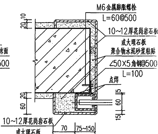
⑤ 花岗石板装修 ⑤a 大理石板装修
