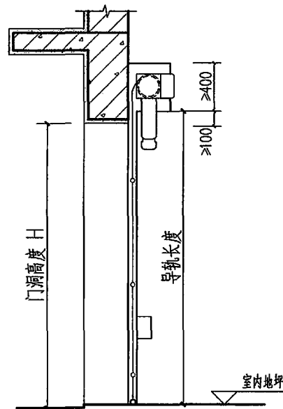
1-1剖面图
