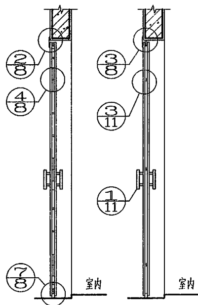
1-1剖面
