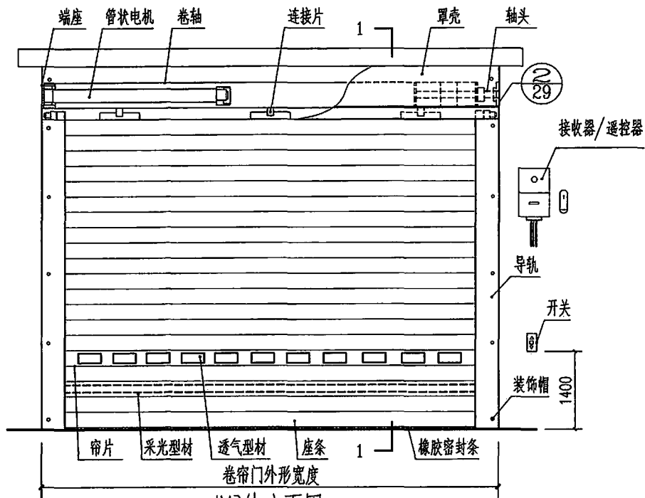
JM3外立面图
