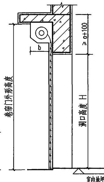
1-1剖面图
