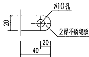
② 锁扣
