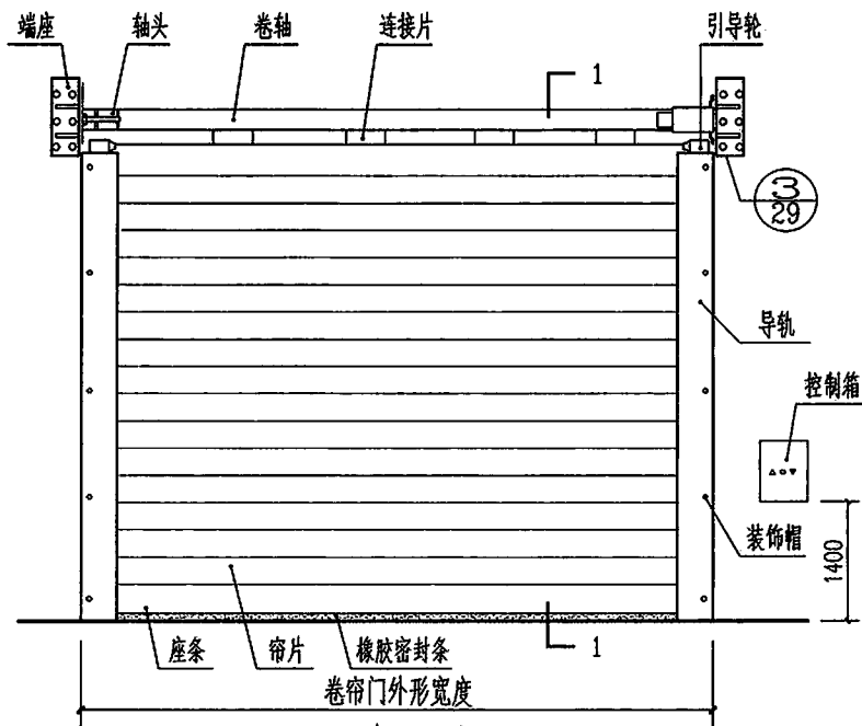
JM4内立面图
