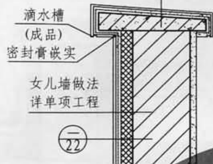
现浇女儿墙压顶详单体设计
