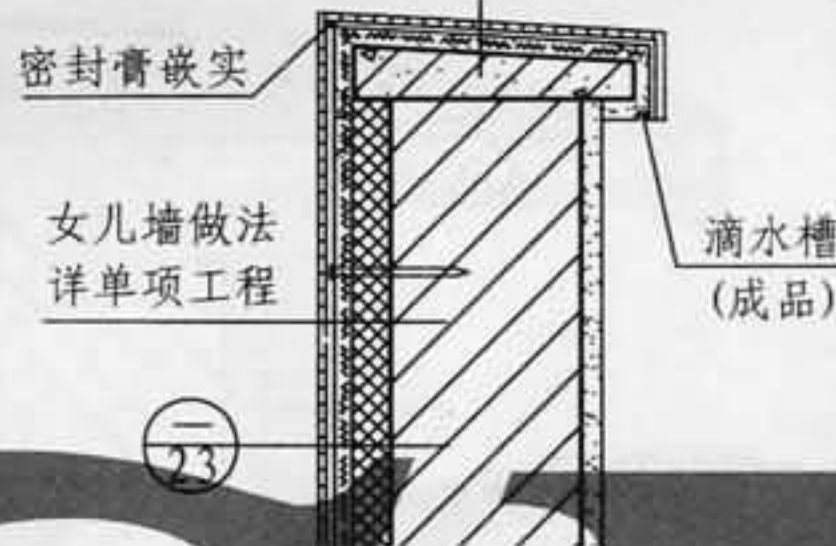
现浇女儿墙压顶详单体设计
