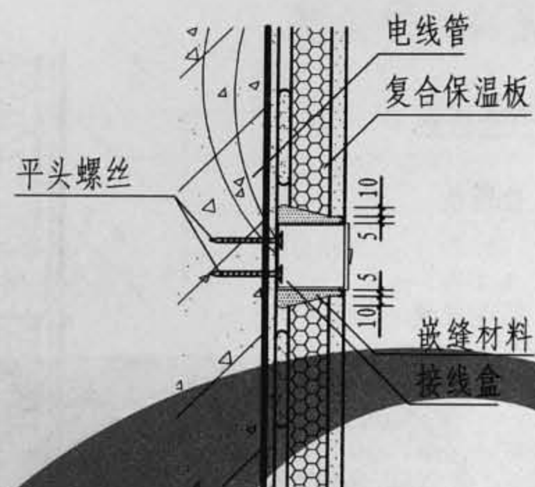
开关盒(一)
