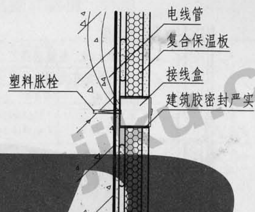
开关盒 (二)
