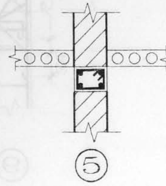
板底圈梁详图(一)
