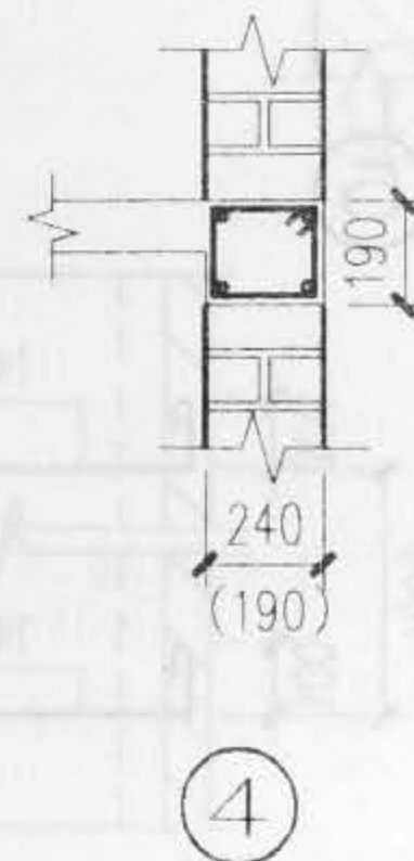
板平圈梁详图(一)
