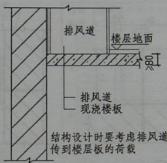
楼层板作为排风道基础
