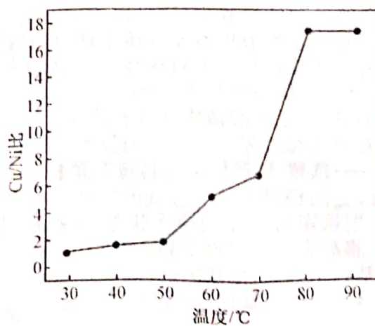
反应温度对滤渣中铜镍比的影响
