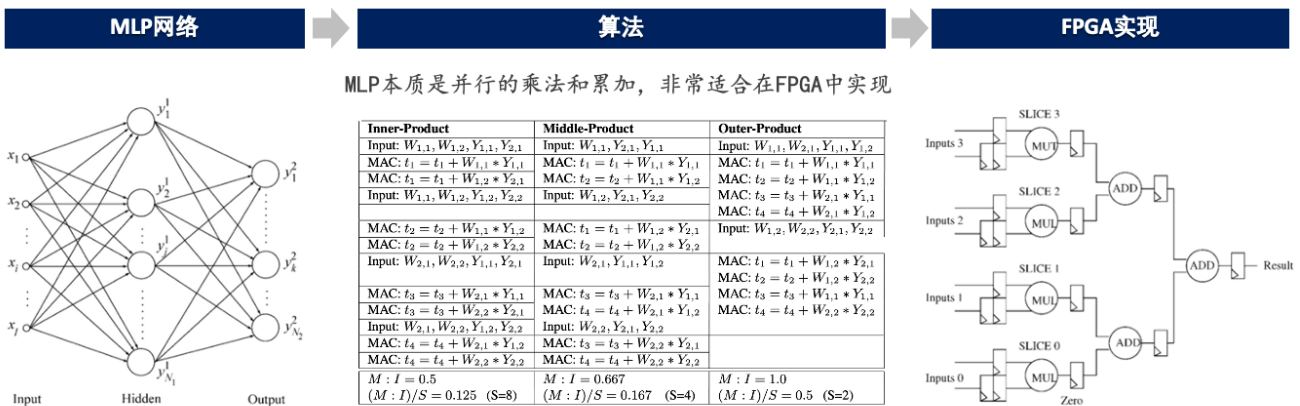
图3：MLP 网络本质是并行的乘法和累加，非常适合在 FPGA 中实现
