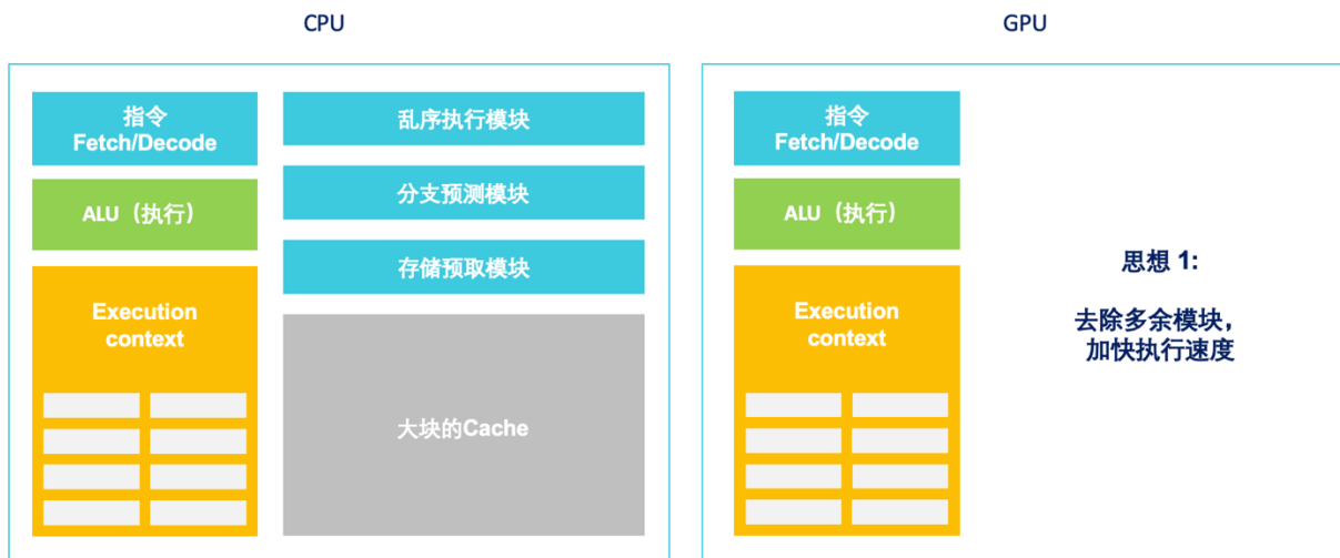
图6: 将 CPU 的核心简化以加快执行速度，是 GPU 设计的思想
